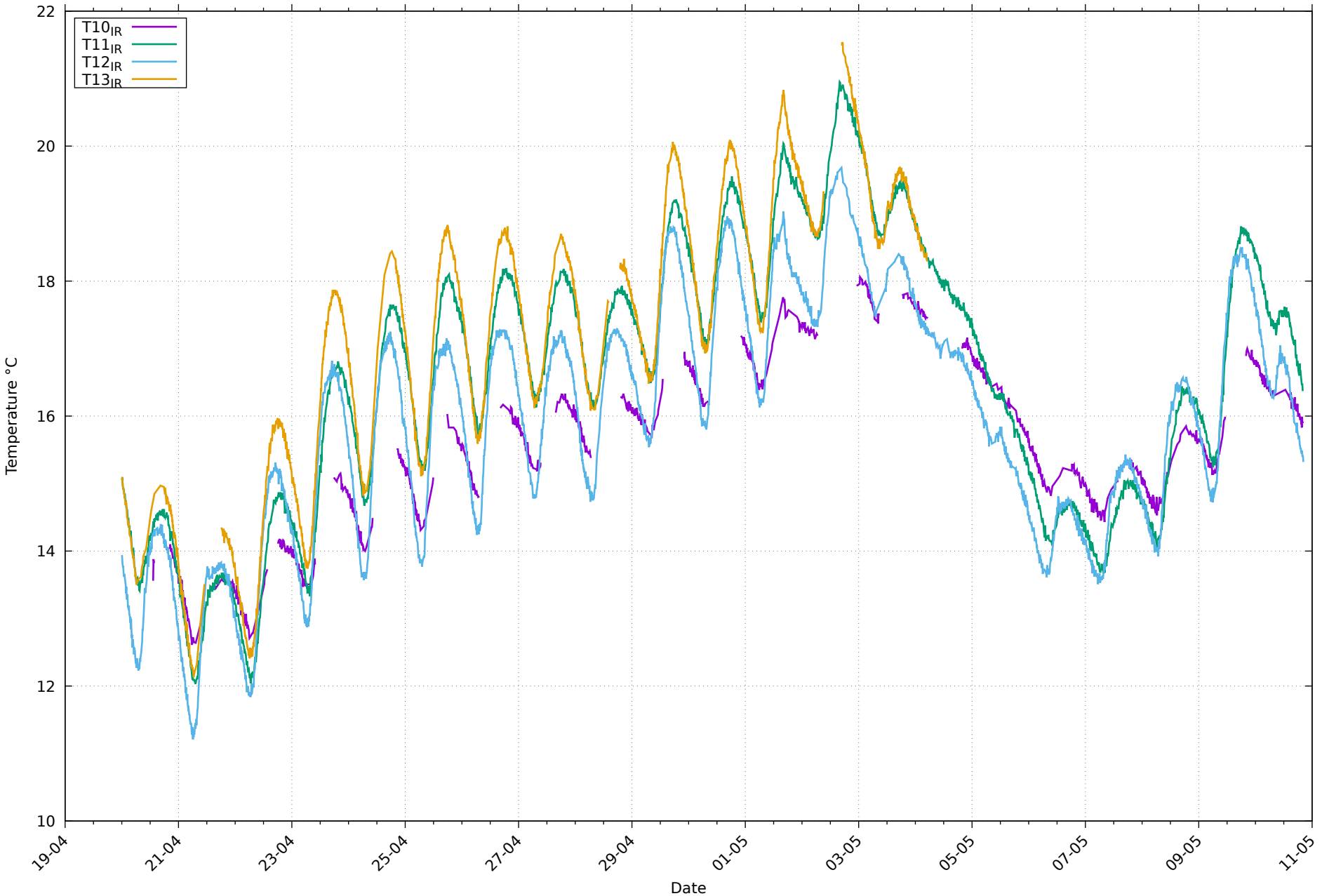
Températures de paroi IR au 10/05/2026
