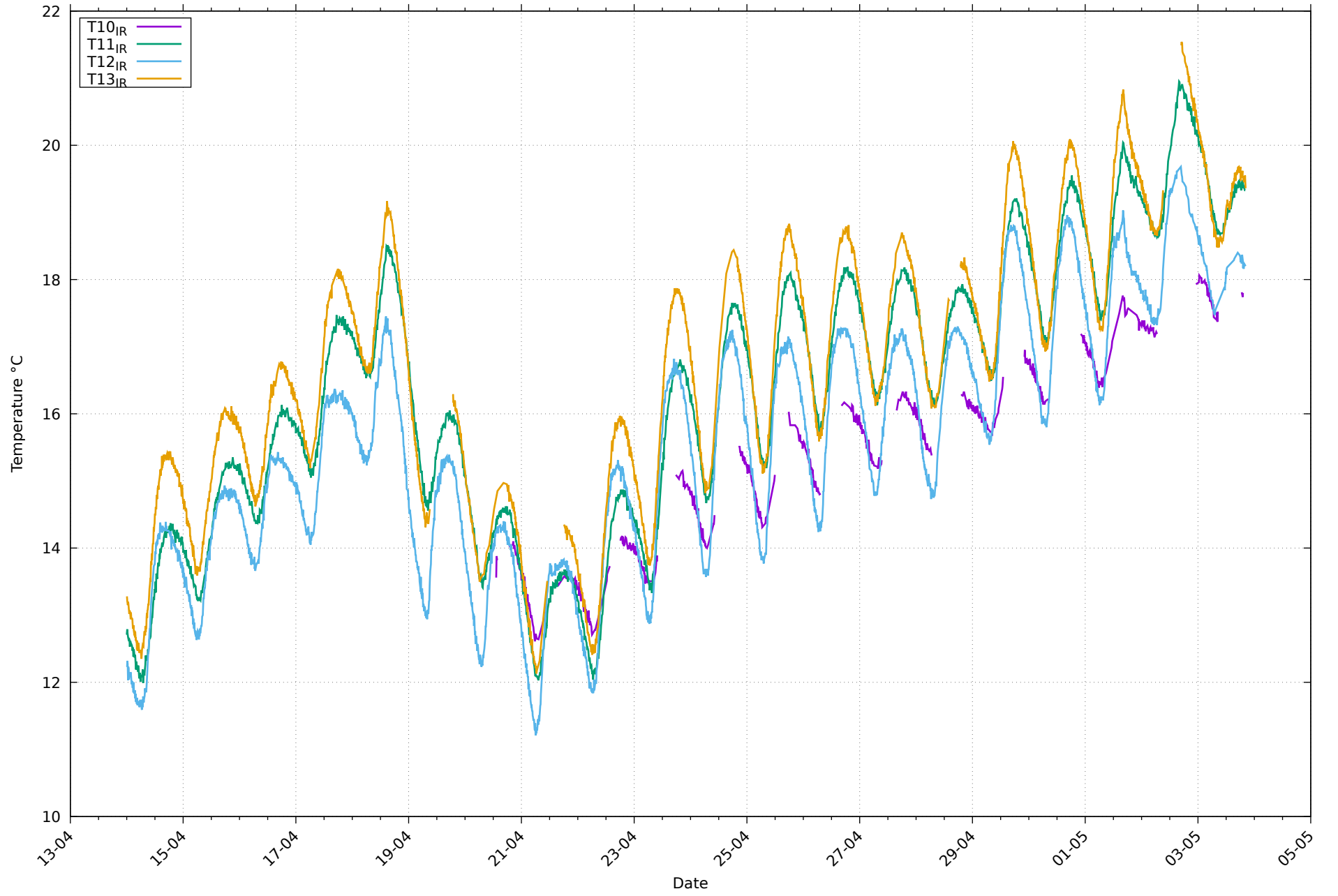
Températures de paroi IR au 03/05/2026
