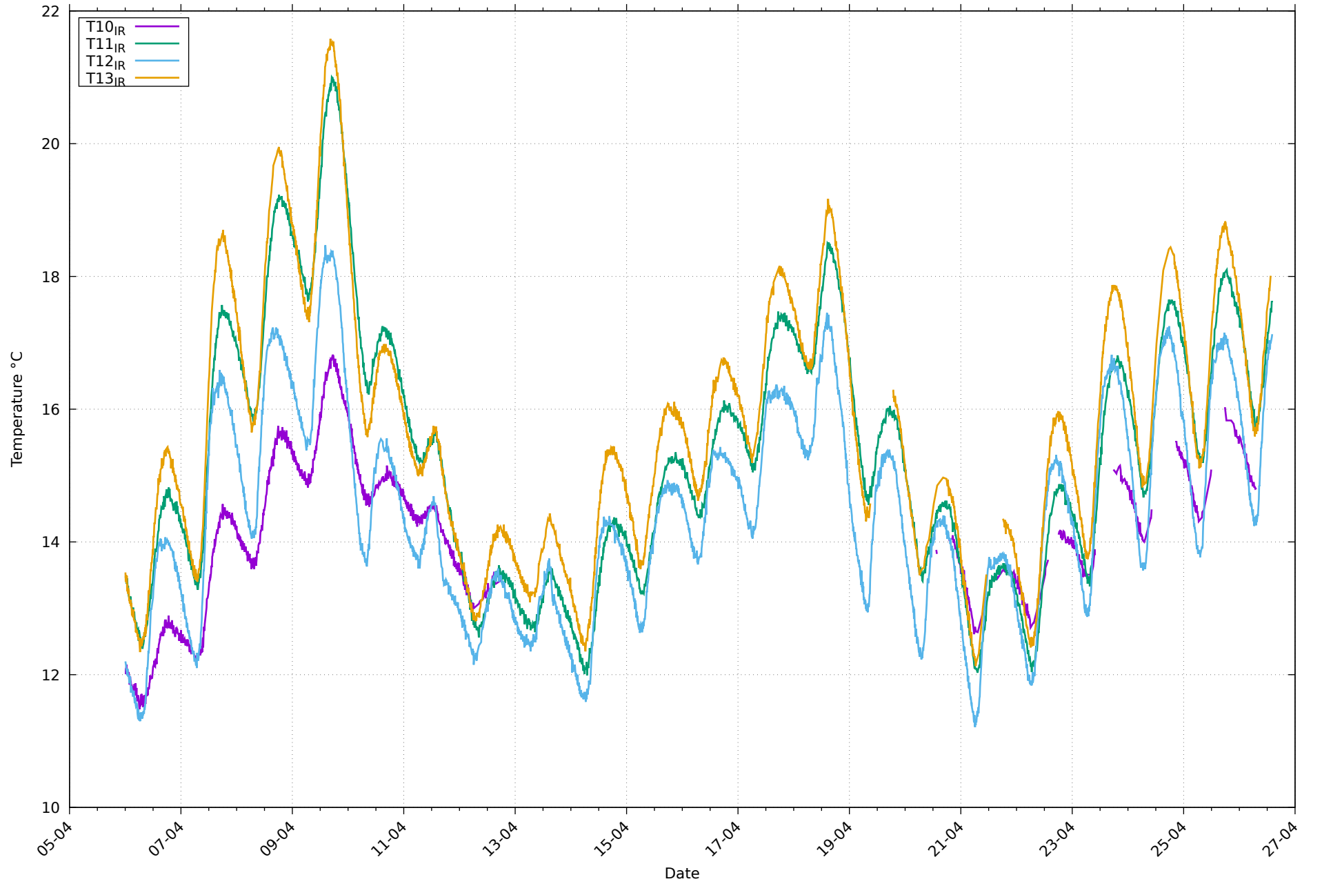
Températures de paroi IR au 26/04/2026
