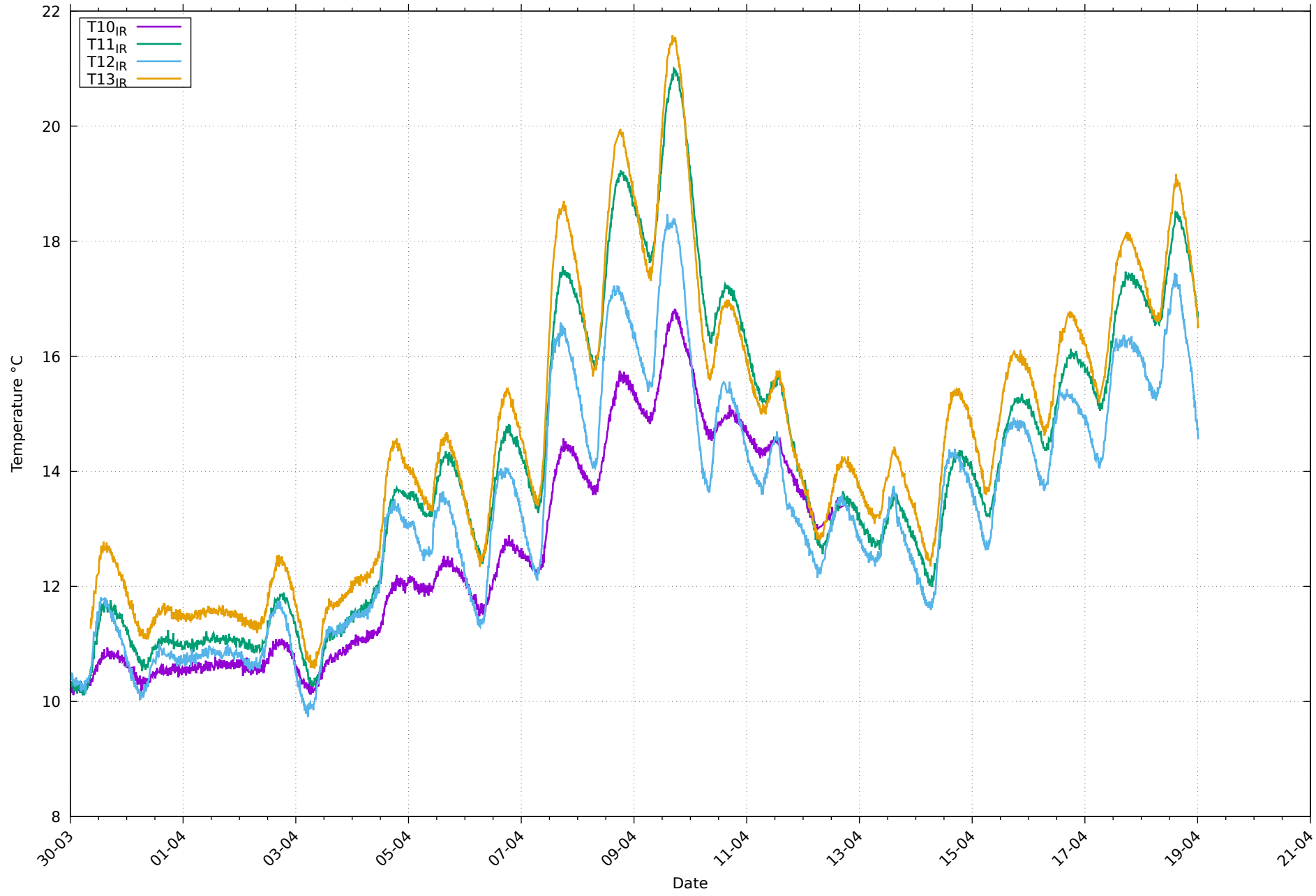
Températures de paroi IR au 19/04/2026
