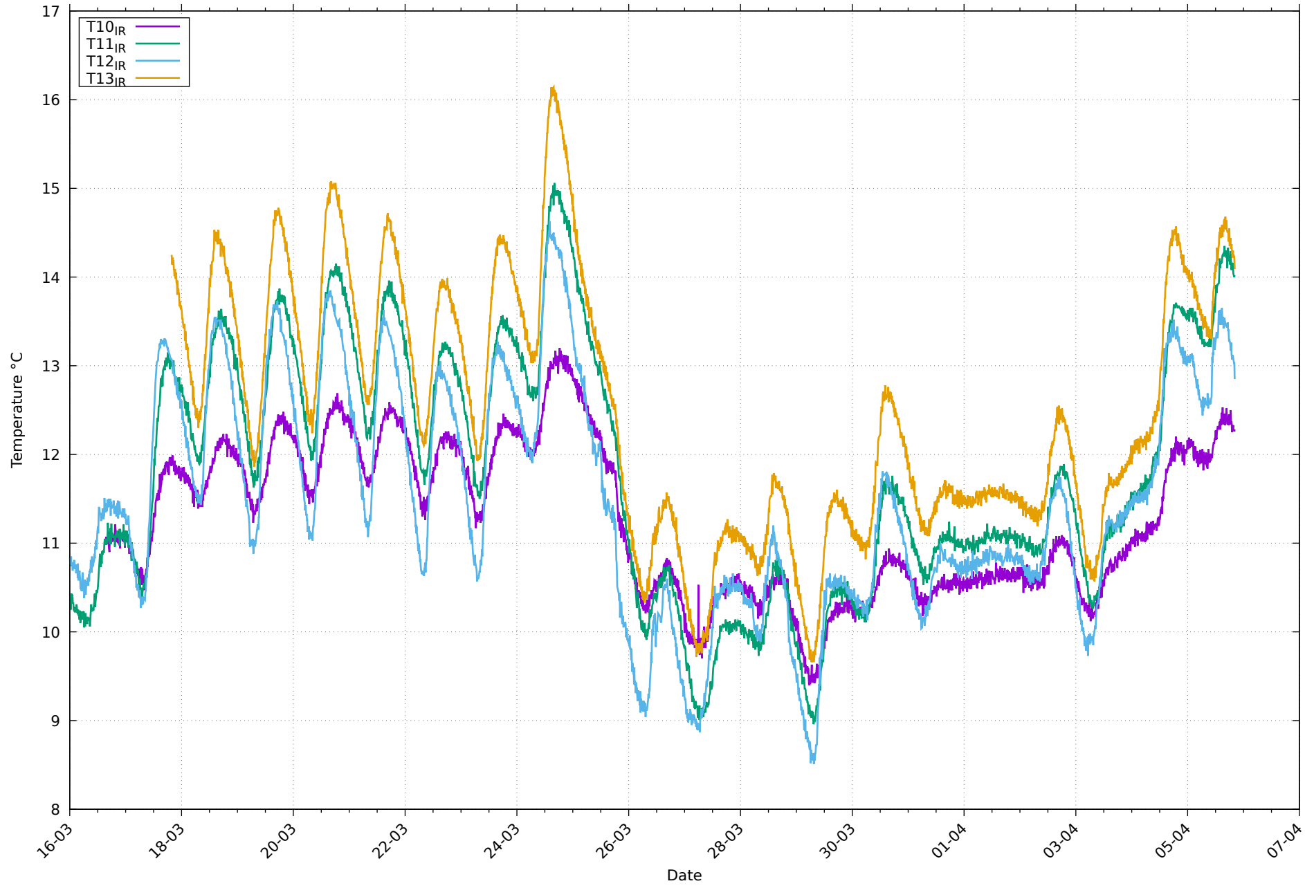
Températures de paroi IR au 05/04/2026
