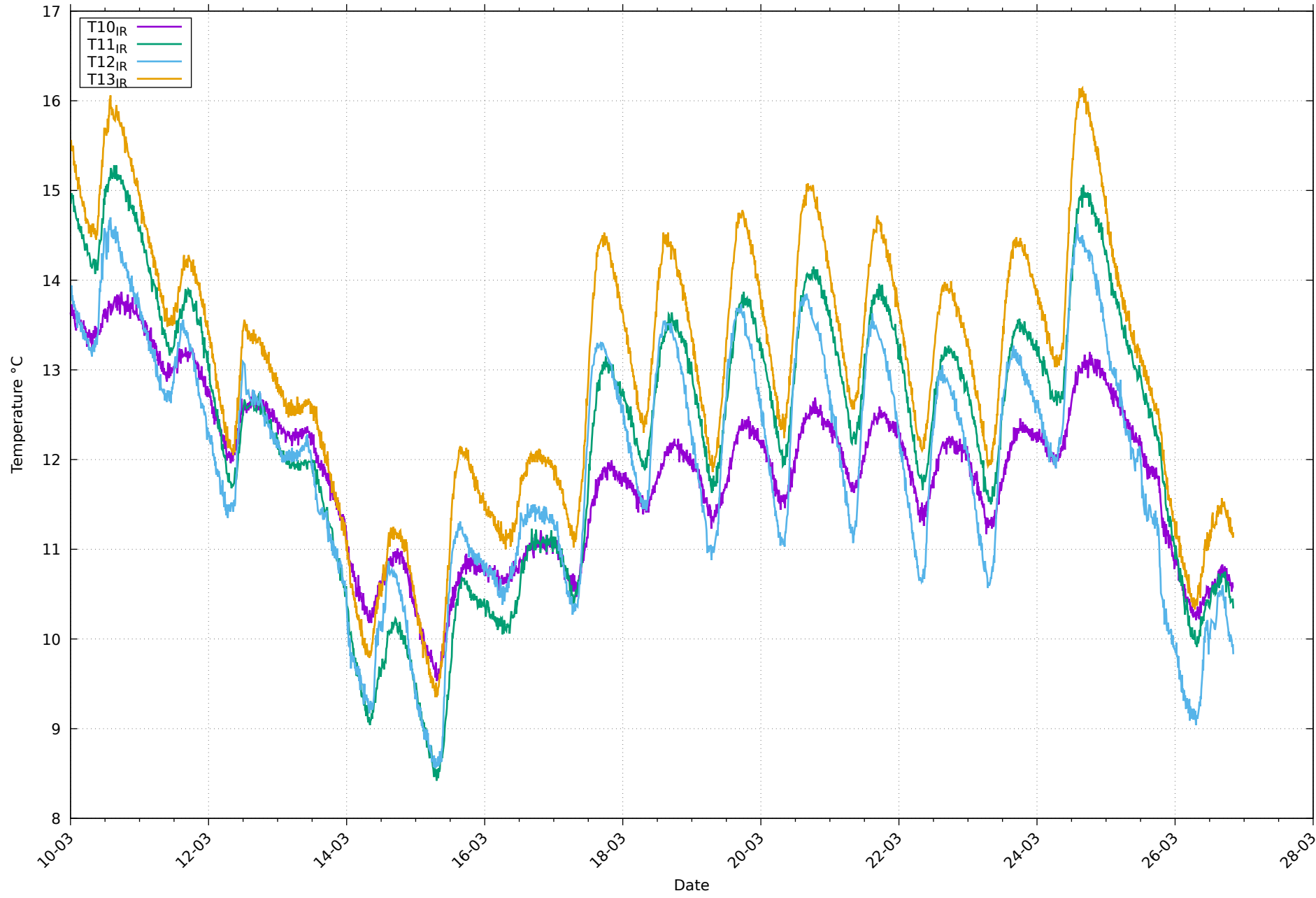
Températures de paroi IR au 29/03/2026
