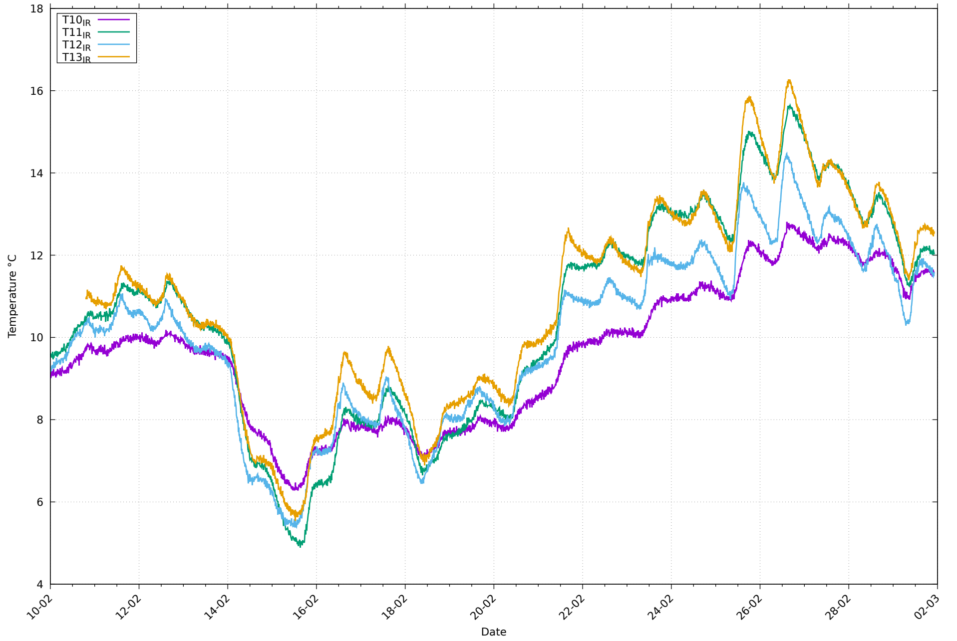
Températures de paroi IR au 01/03/2026
