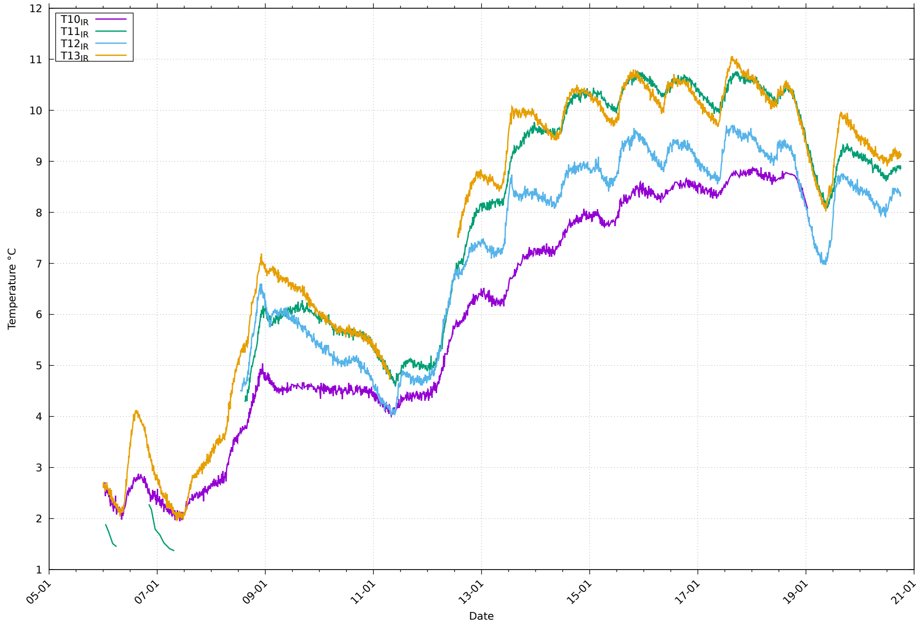
Températures de paroi IR au 25/01/2026
