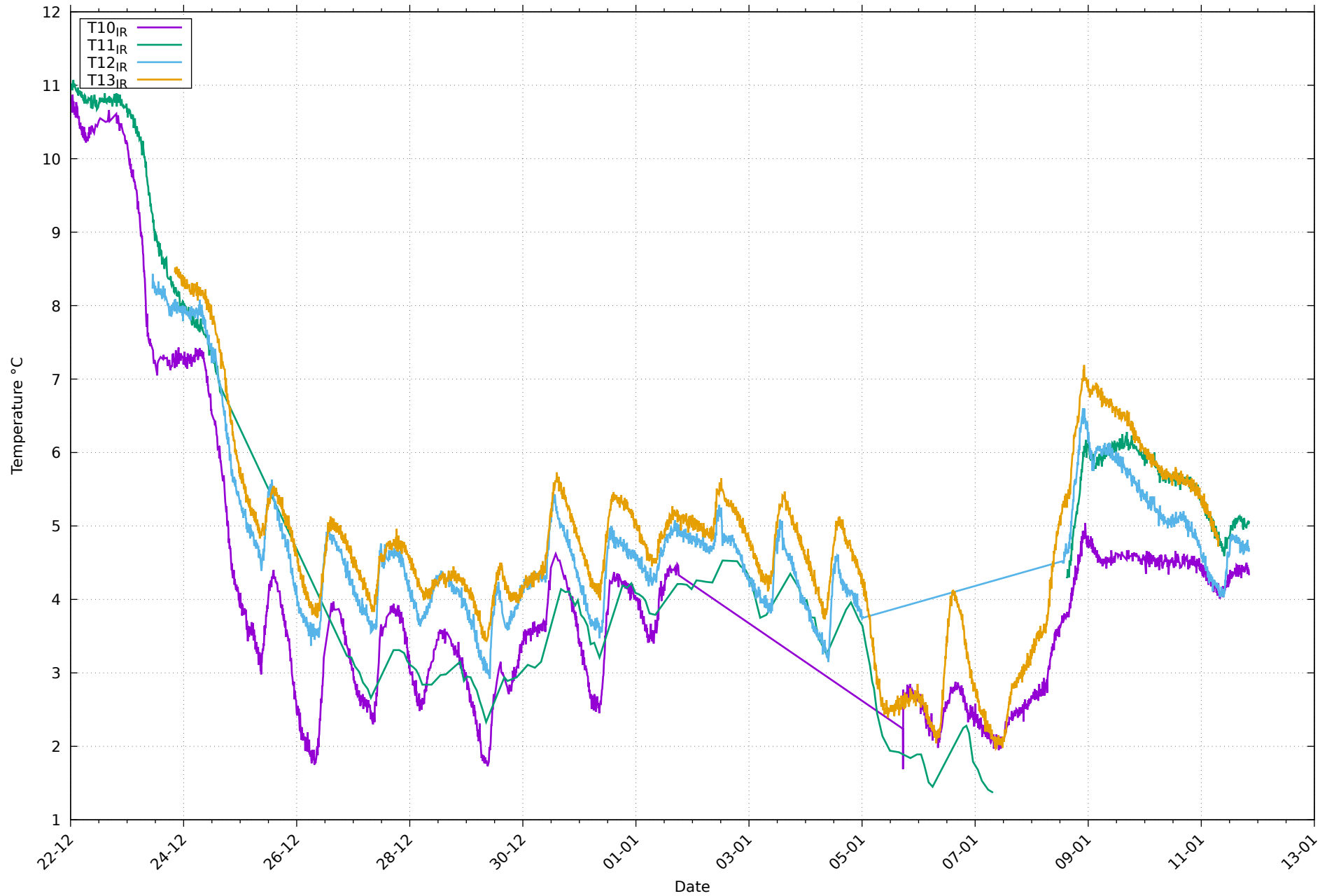
Températures de paroi IR au 11/01/2026
