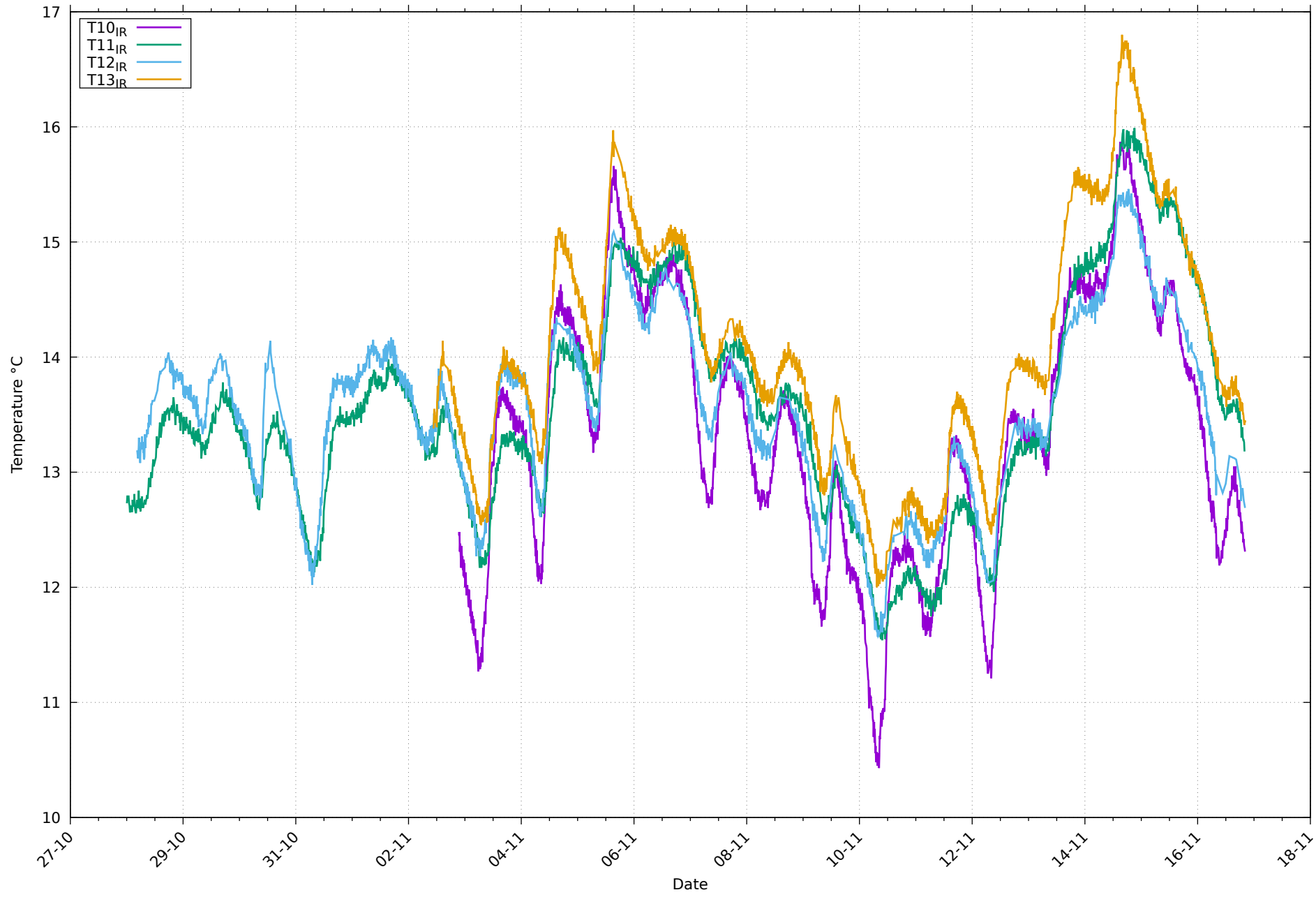
Températures de paroi IR au 16/11/2025
