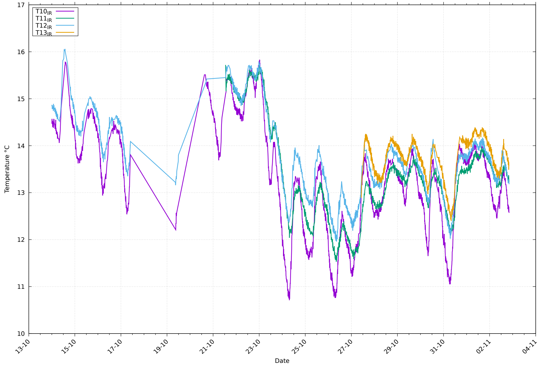
Températures de paroi IR au 02/11/2025
