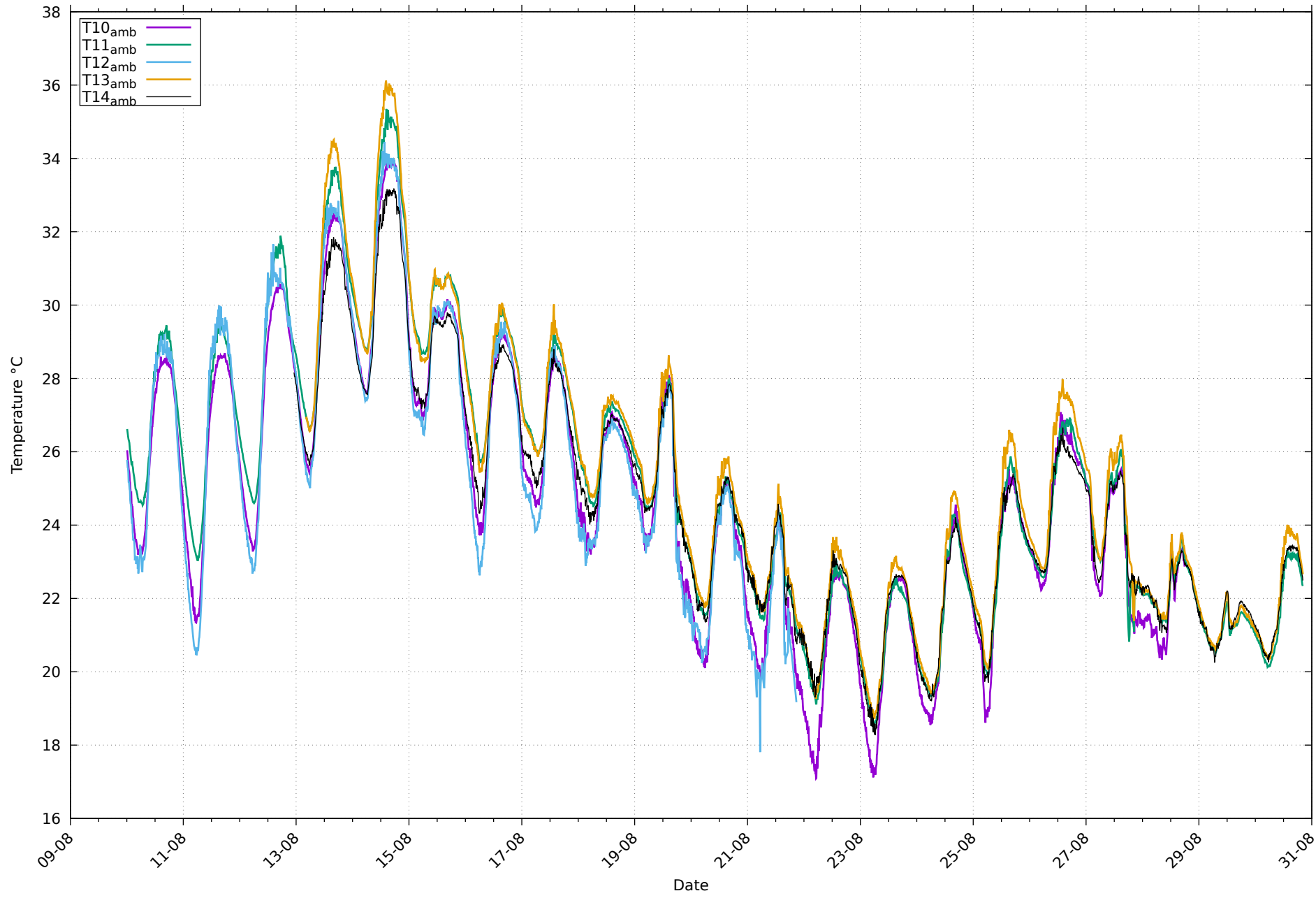
Températures ambiantes au 30/08/2026
