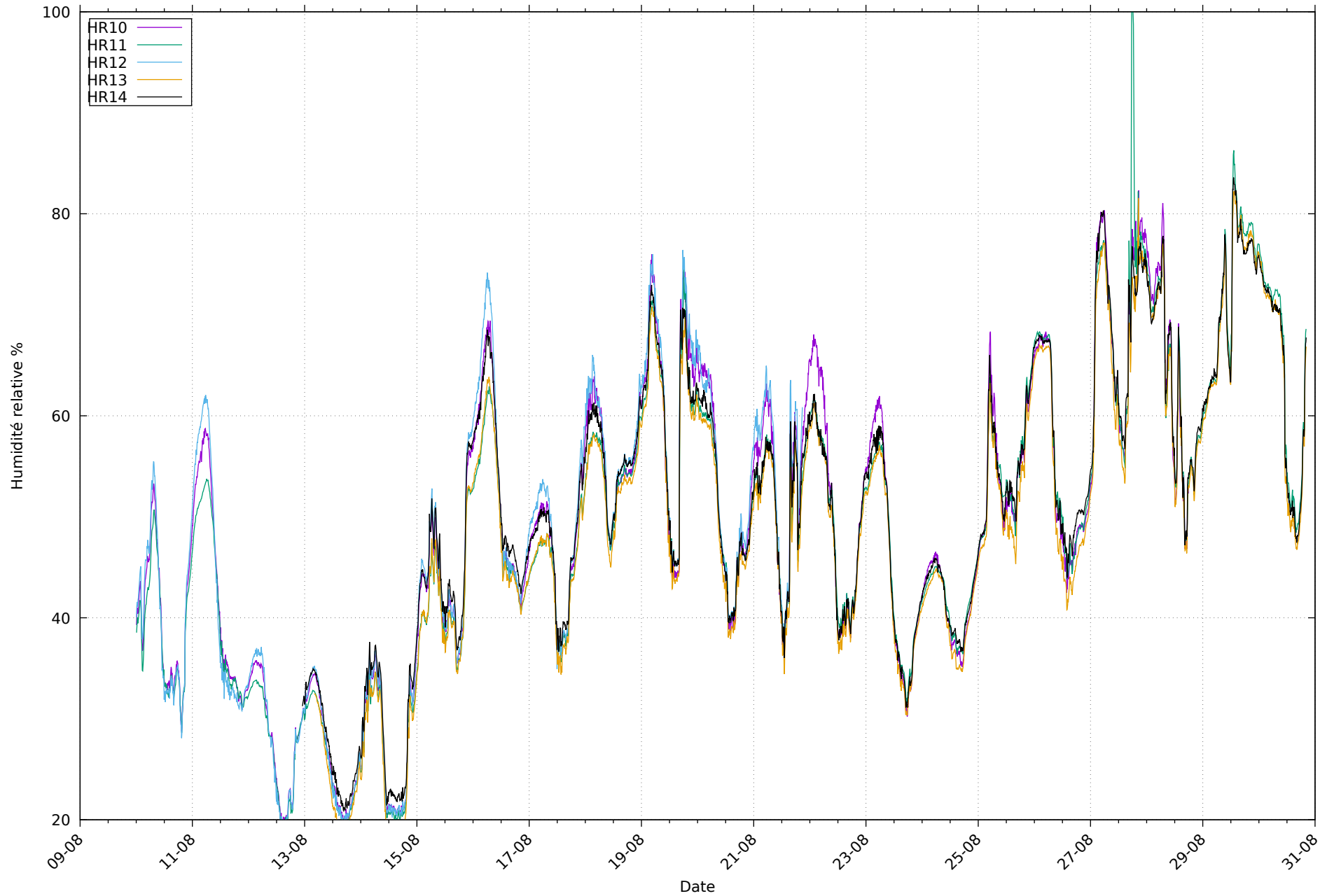
Humidités au 30/08/2026
