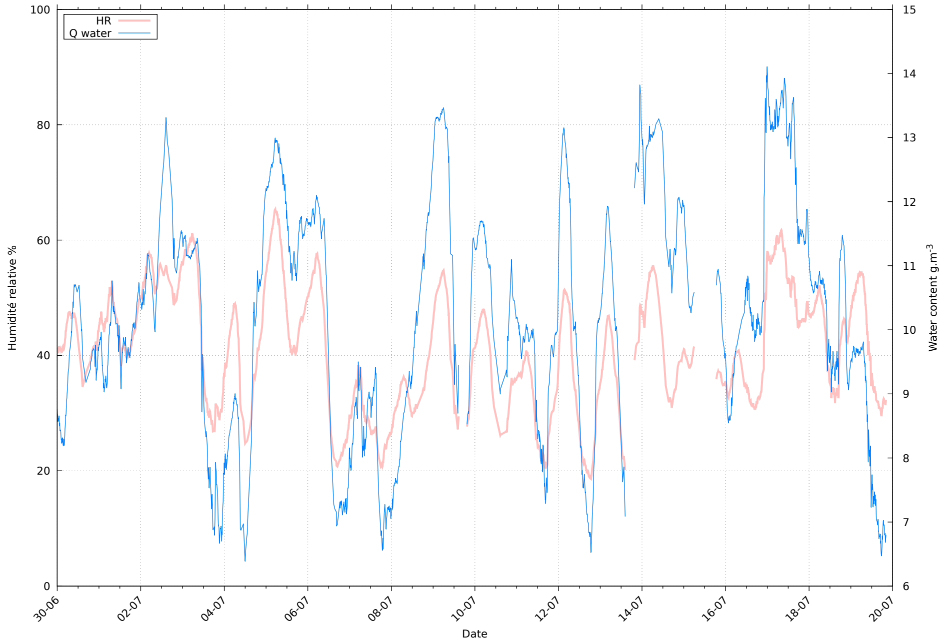
Humidité au 19/07/2026 pour RHT13
