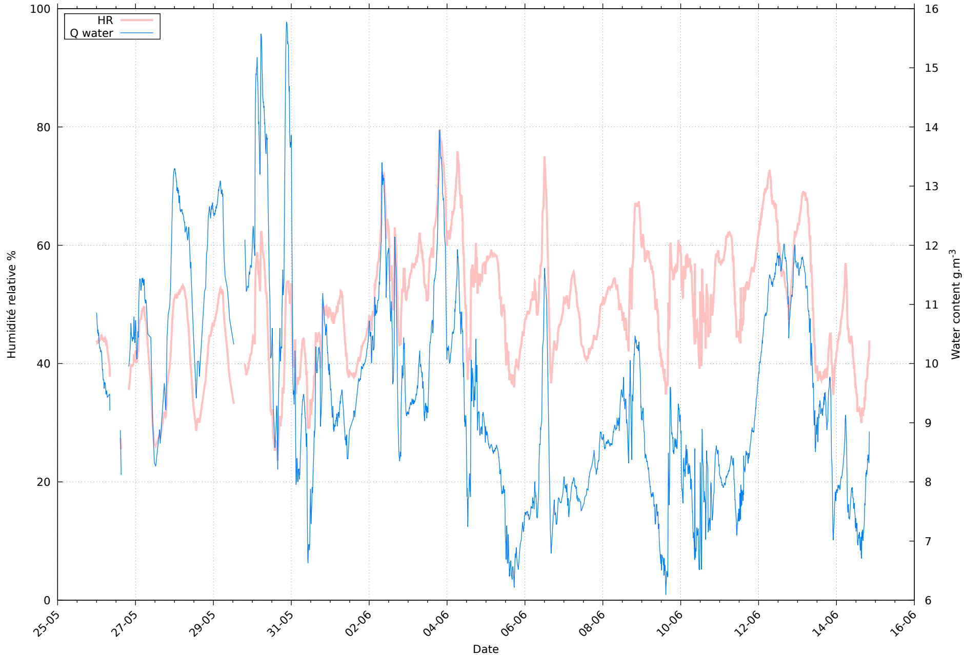
Humidité au 14/06/2026 pour RHT13
