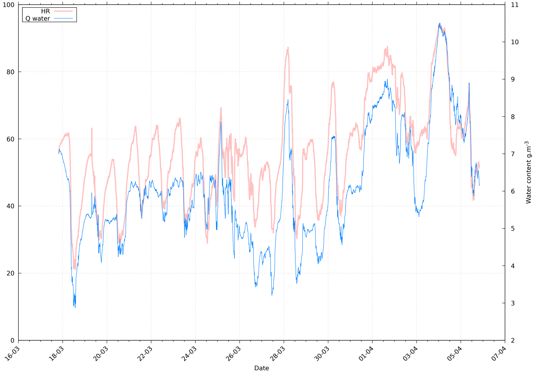
Humidité au 05/04/2026 pour RHT13
