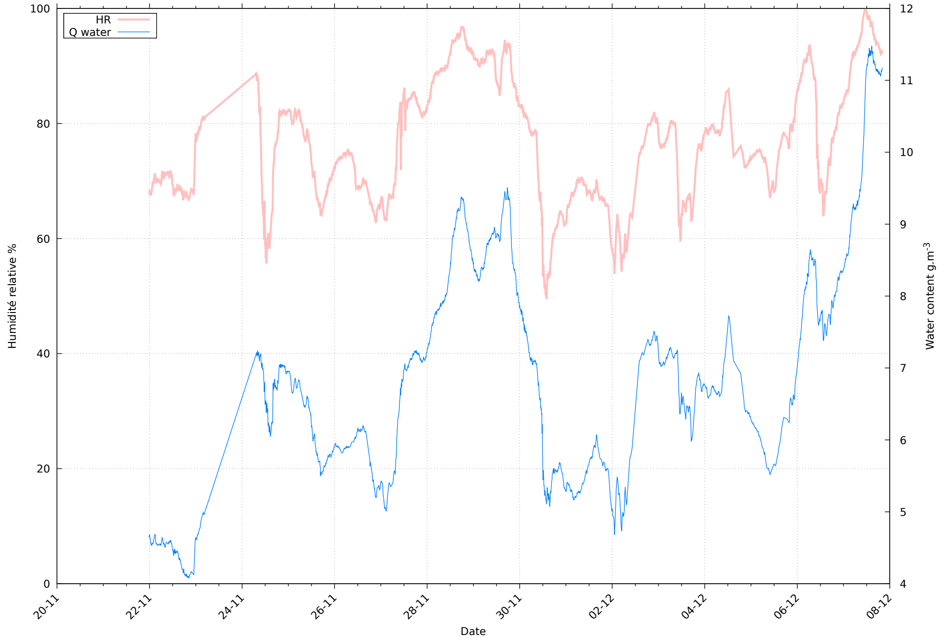
Humidité au 07/12/2025 pour RHT13
