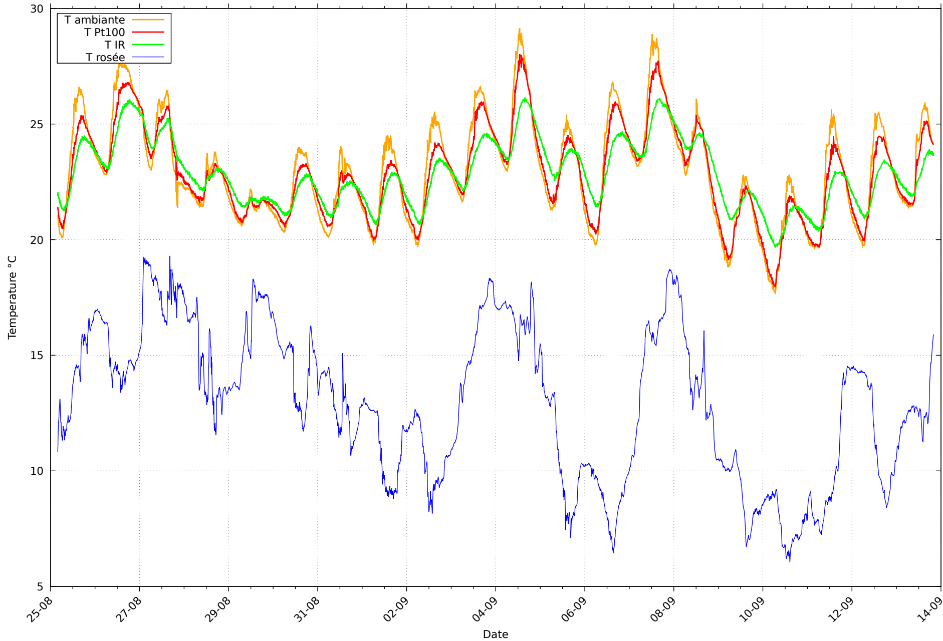
Température et rosée au 13/09/2026 pour RHT13
