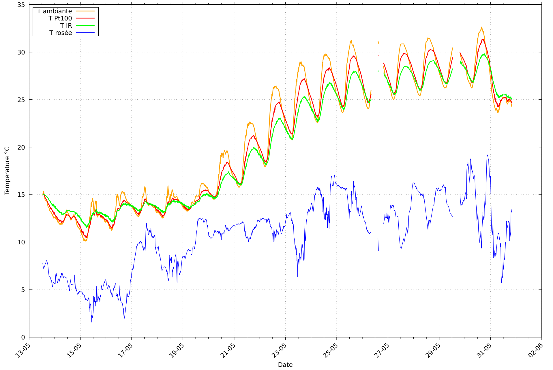
Température et rosée au 31/05/2026 pour RHT13
