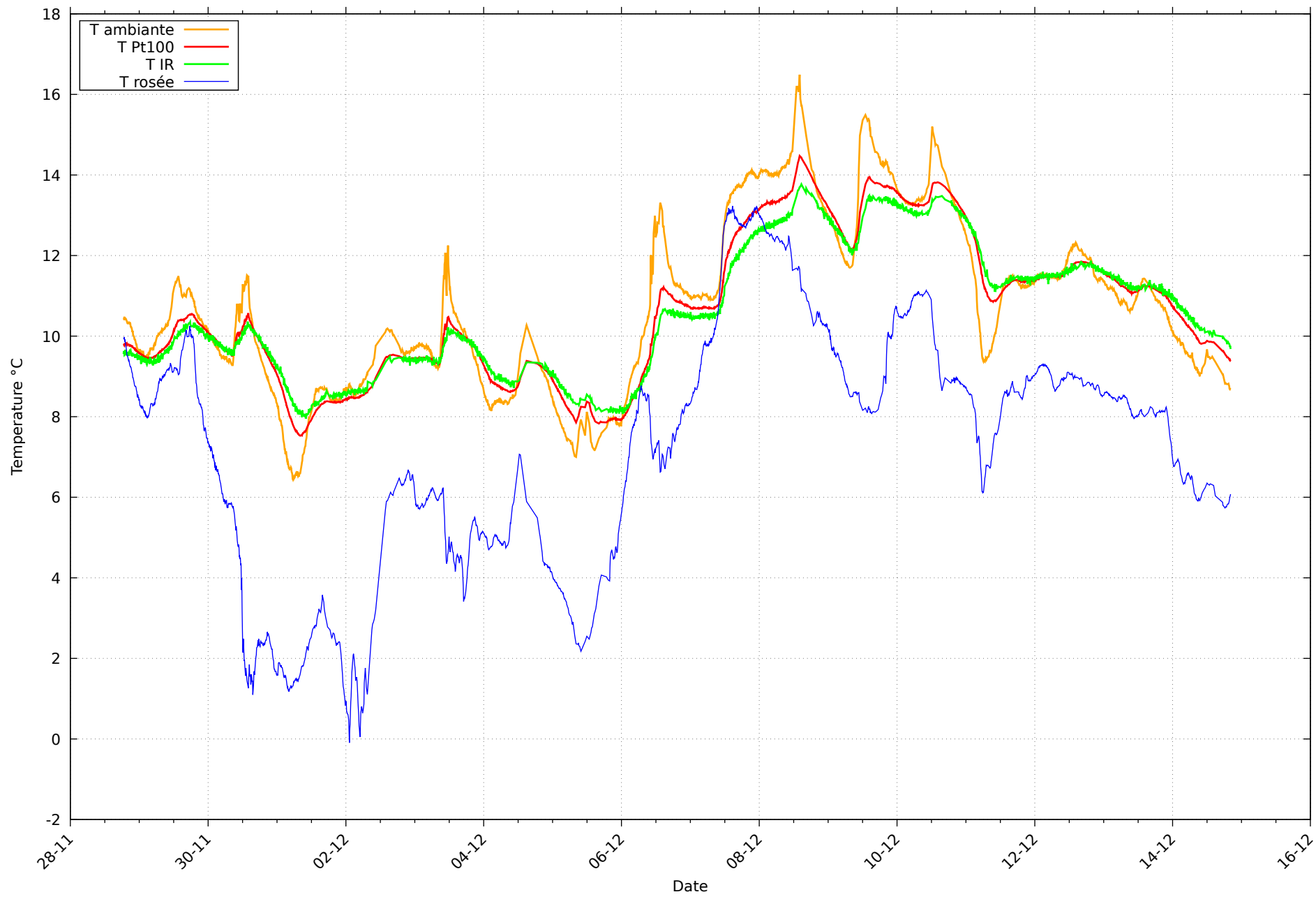
Température et rosée au 14/12/2025 pour RHT13
