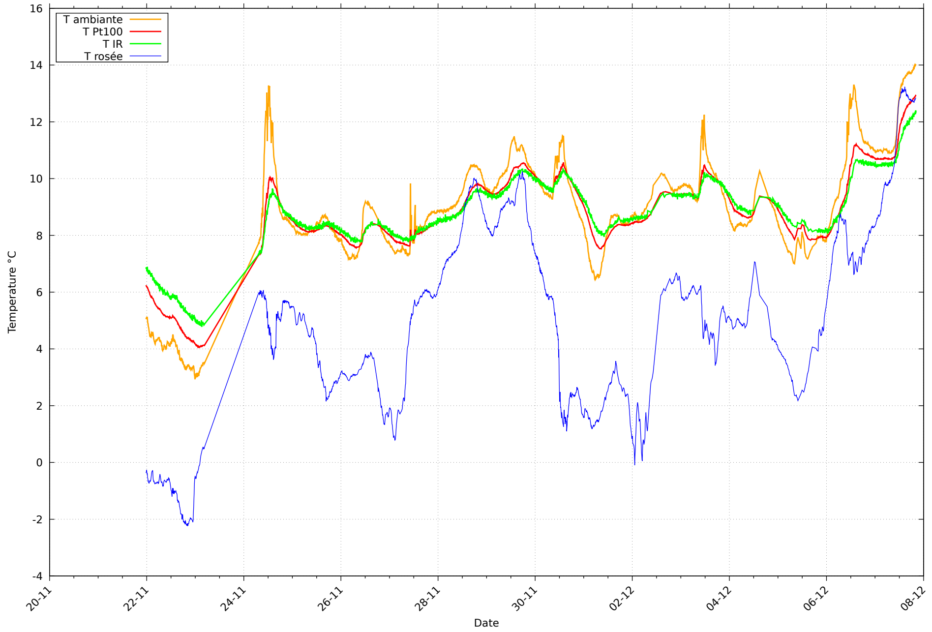
Température et rosée au 07/12/2025 pour RHT13
