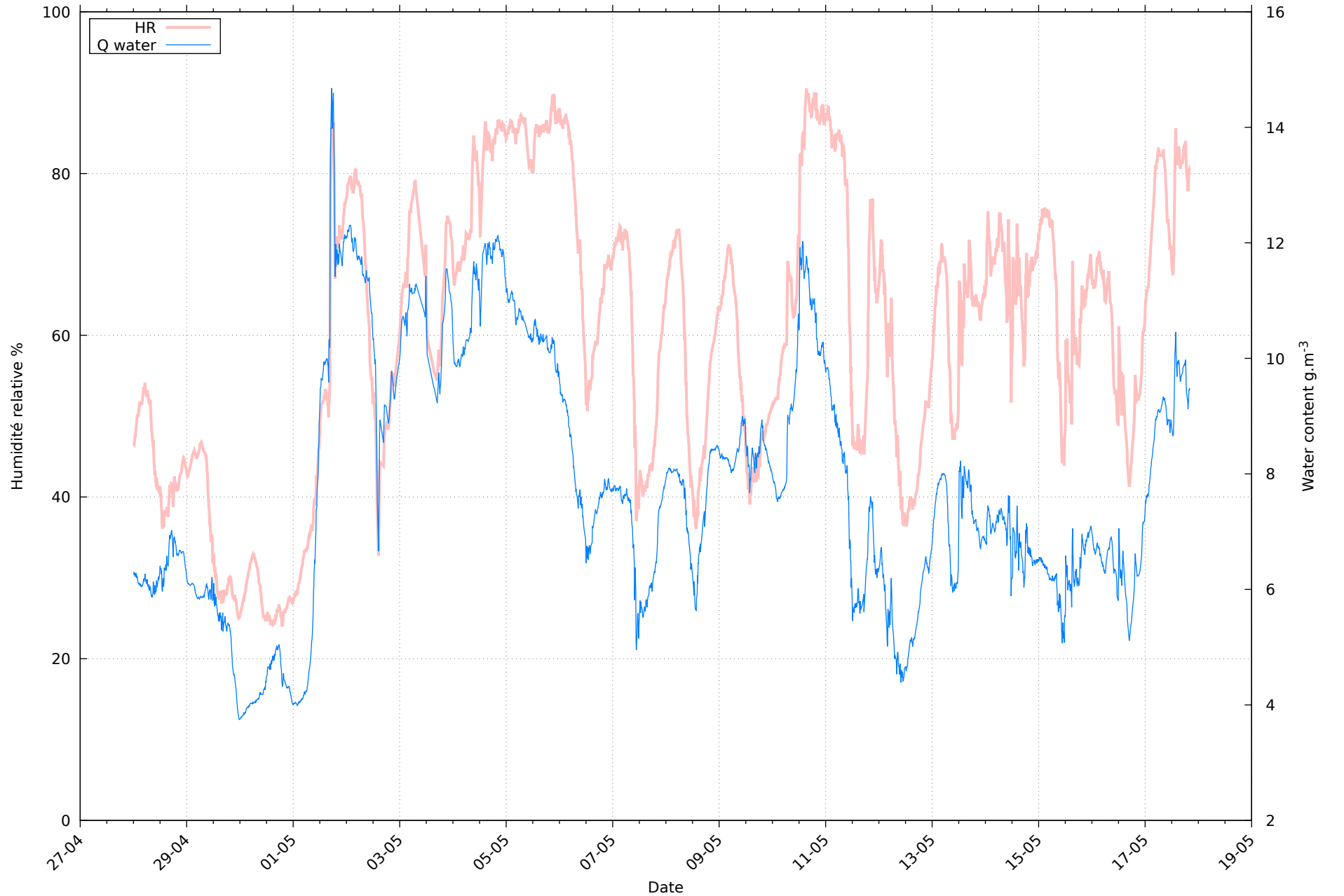
Humidité au 17/05/2026 pour RHT12
