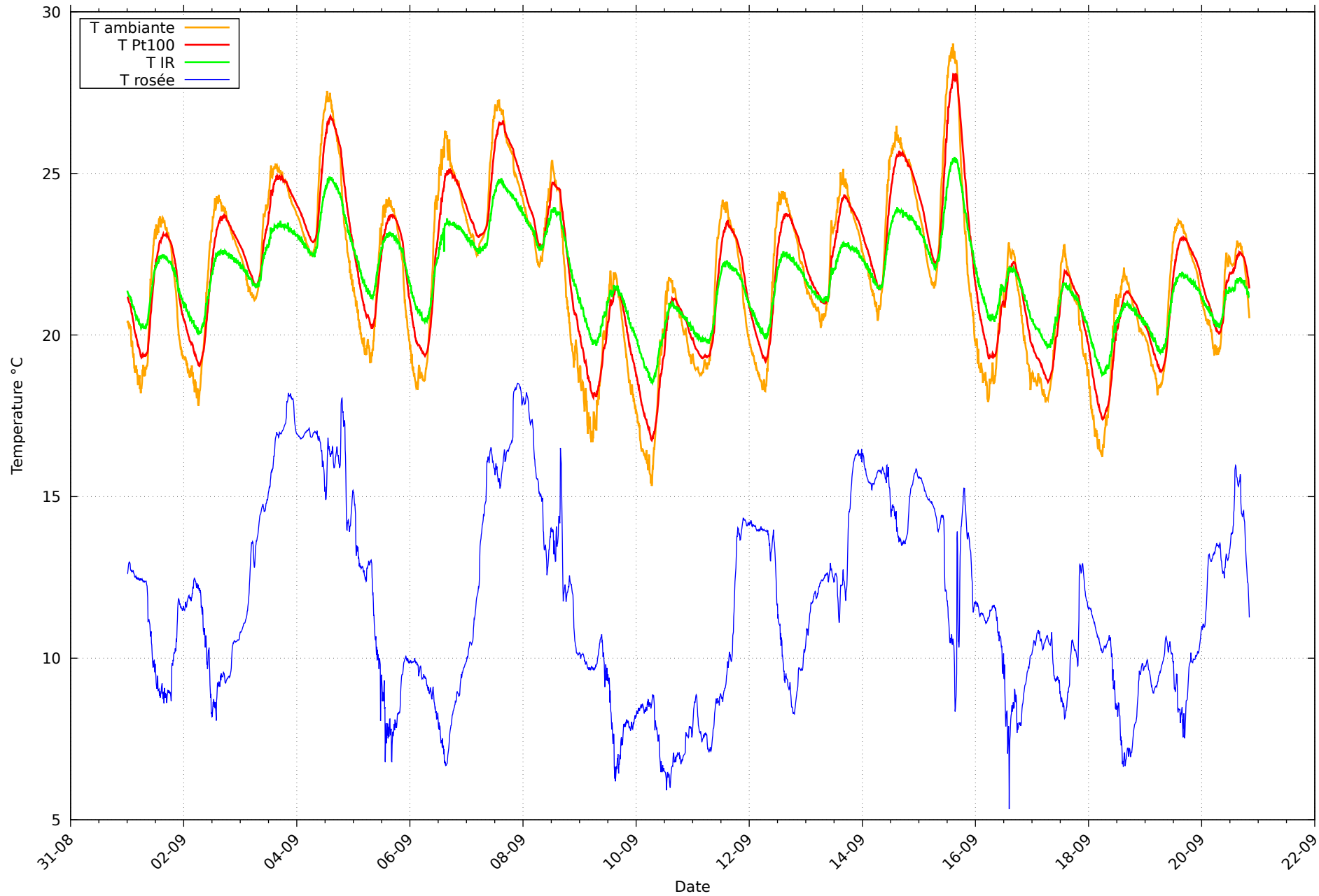
Température et rosée au 20/09/2026 pour RHT12
