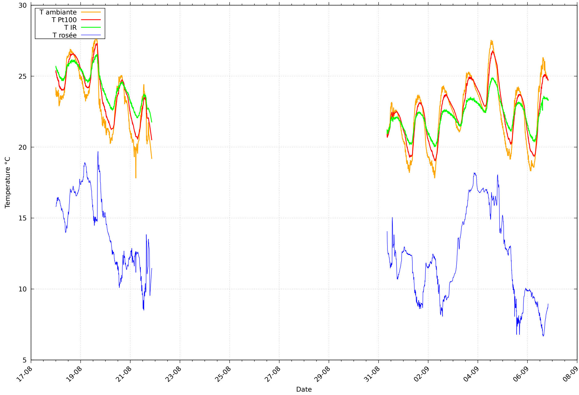
Température et rosée au 06/09/2026 pour RHT12
