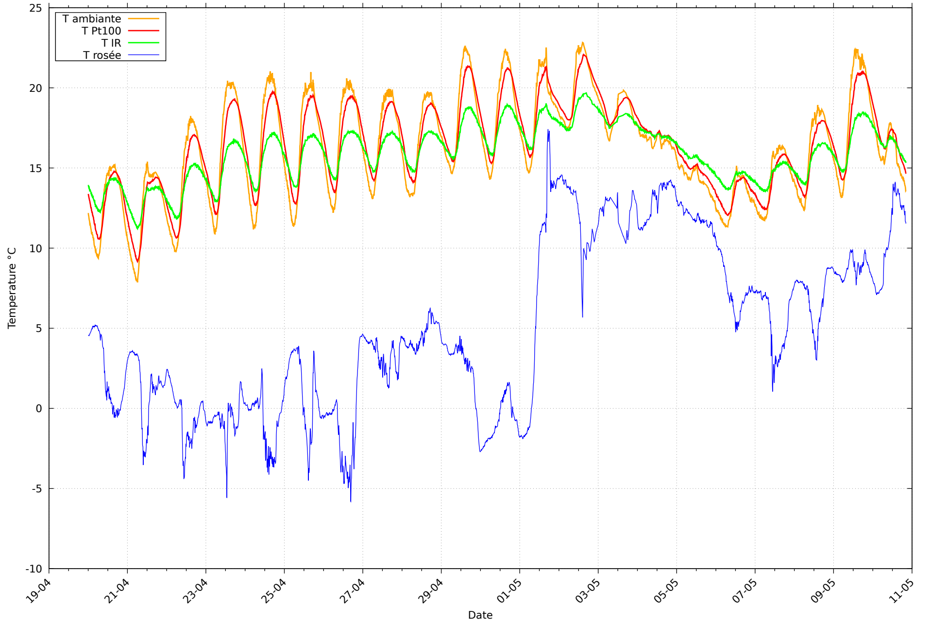
Température et rosée au 10/05/2026 pour RHT12
