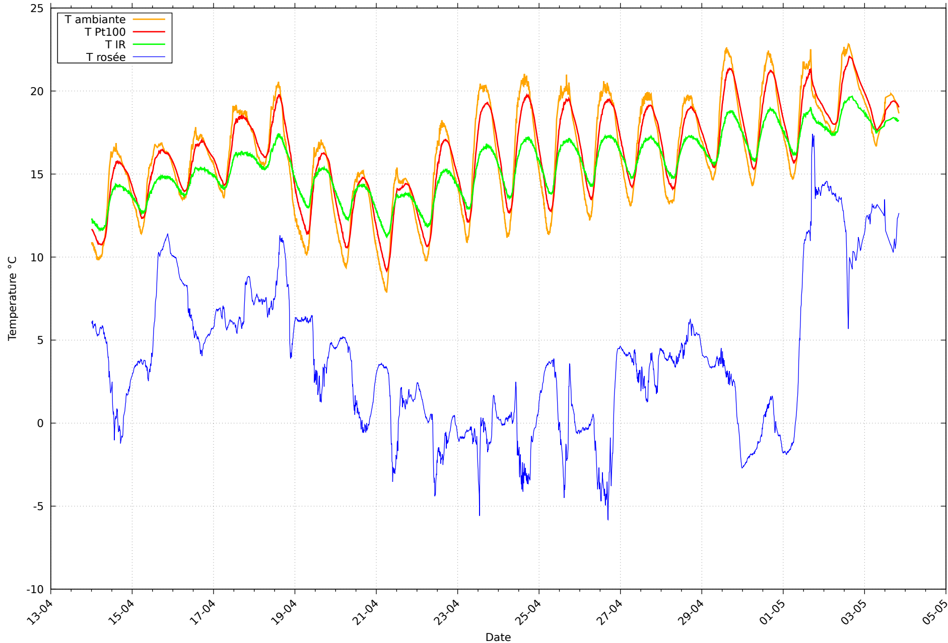
Température et rosée au 03/05/2026 pour RHT12
