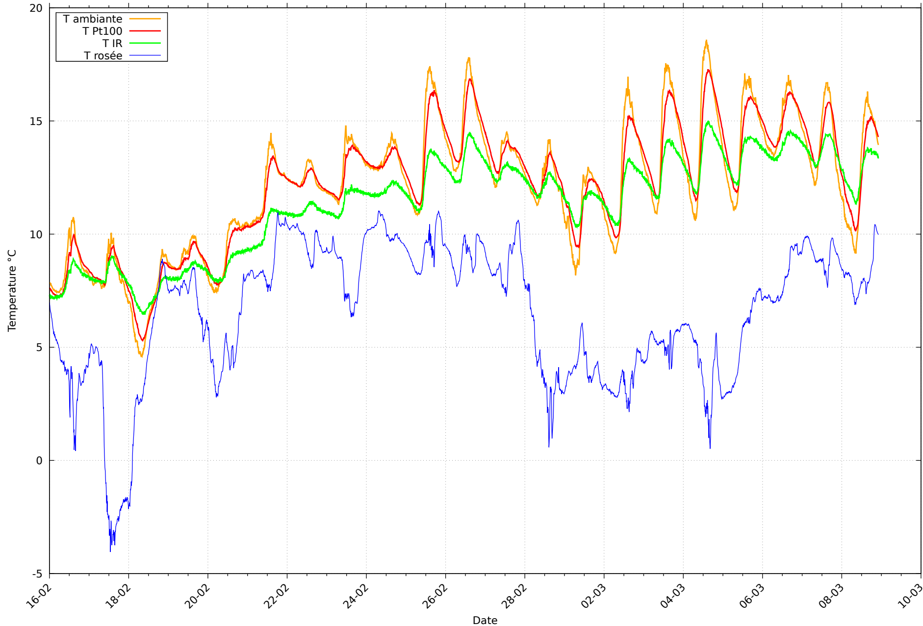
Température et rosée au 08/03/2026 pour RHT12
