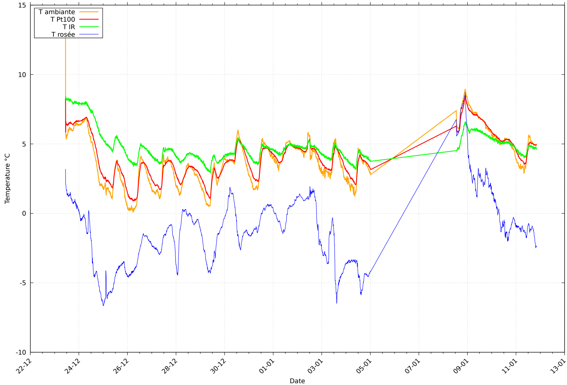
Température et rosée au 11/01/2026 pour RHT12
