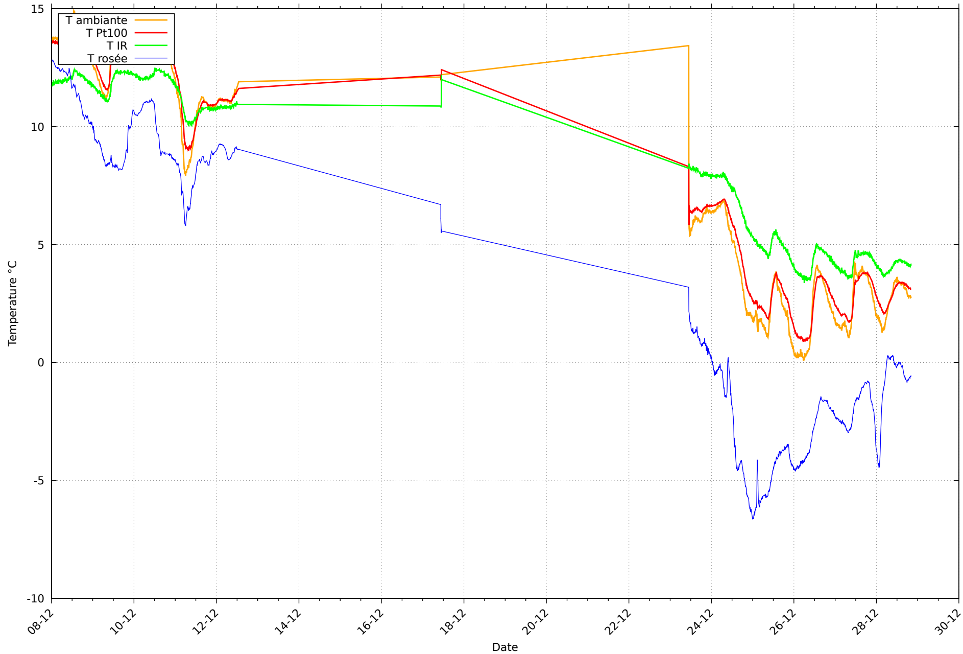
Température et rosée au 28/12/2025 pour RHT12
