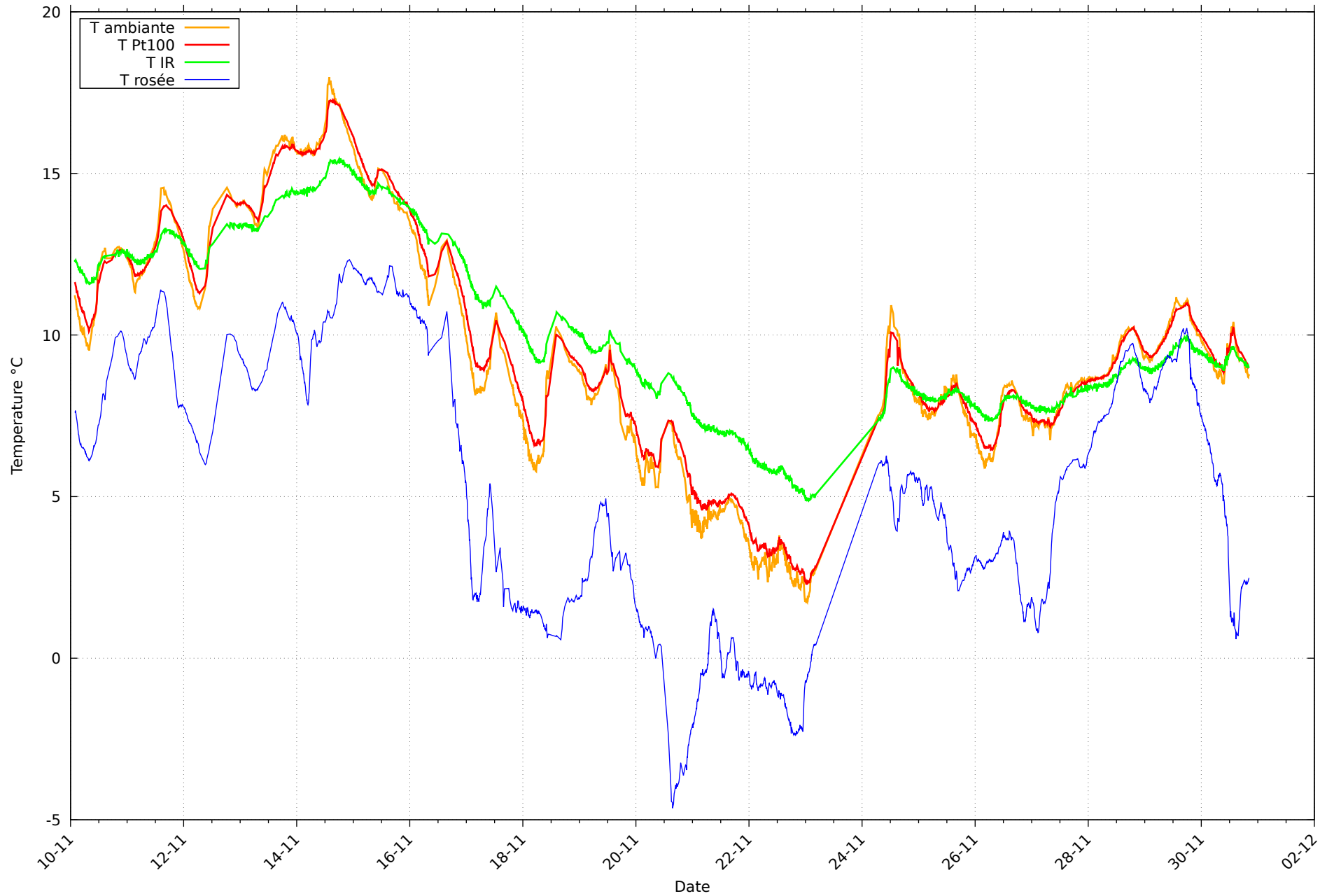
Température et rosée au 30/11/2025 pour RHT12
