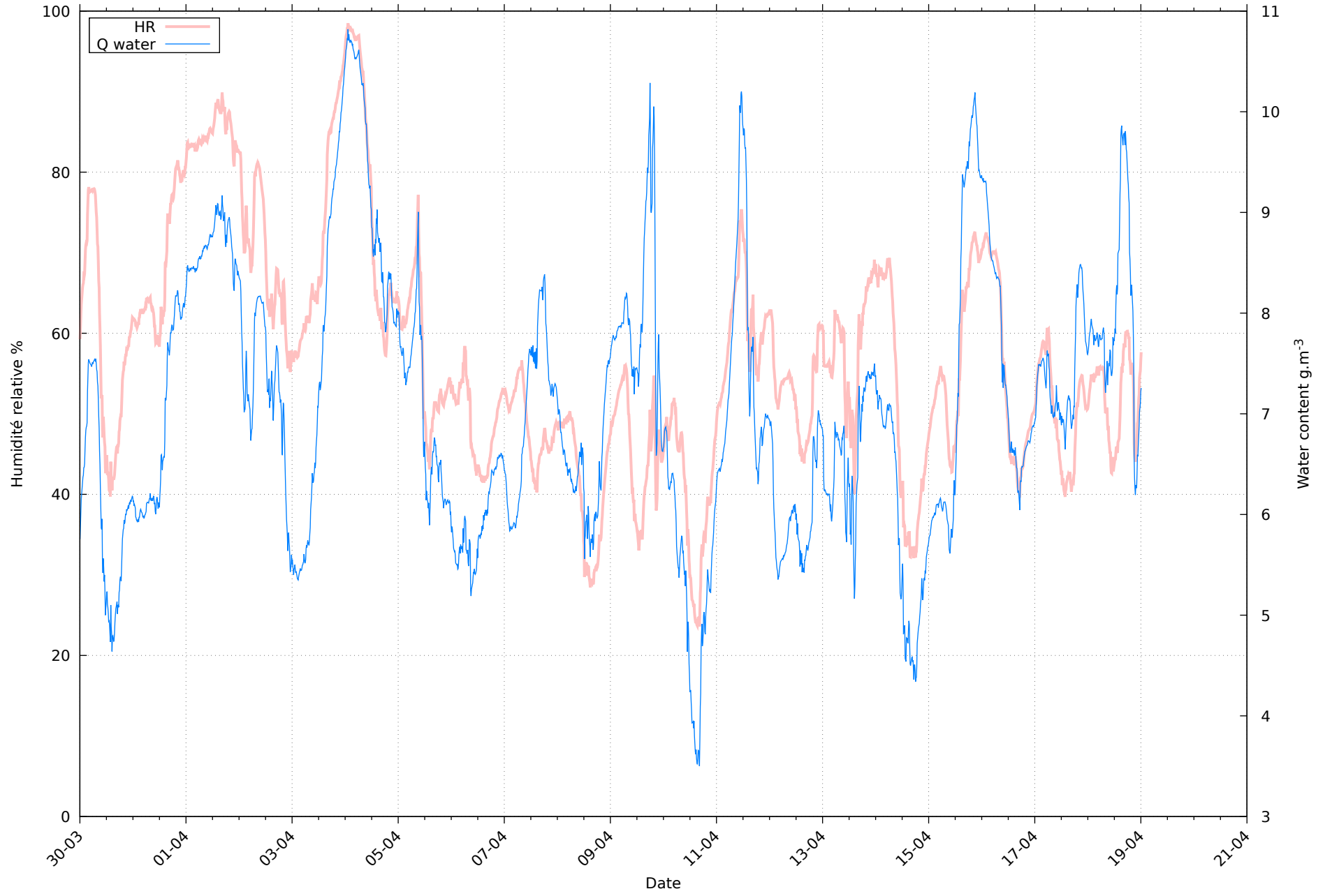
Humidité au 19/04/2026 pour RHT11
