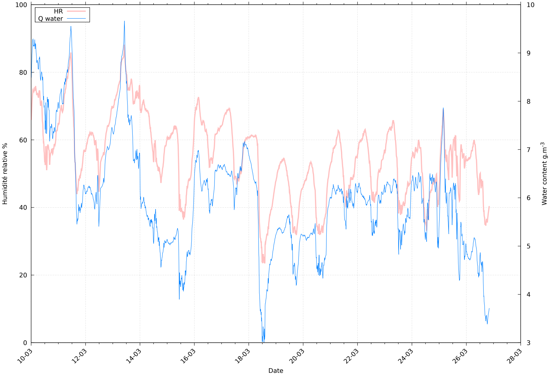
Humidité au 29/03/2026 pour RHT11
