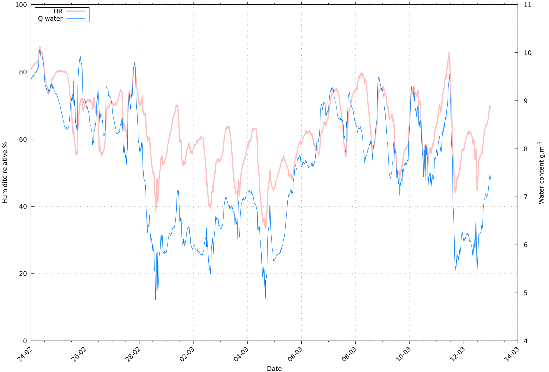
Humidité au 15/03/2026 pour RHT11
