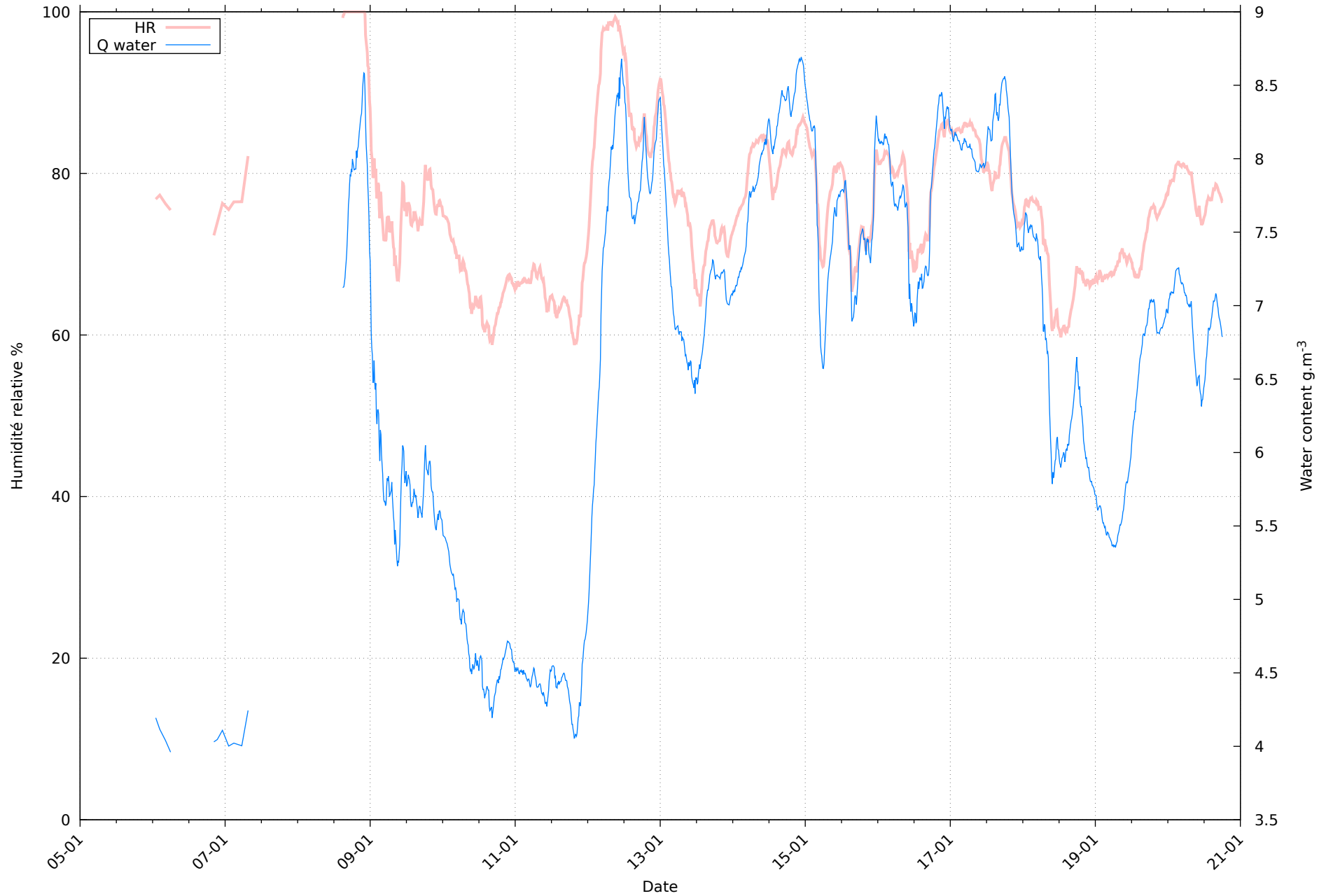
Humidité au 25/01/2026 pour RHT11
