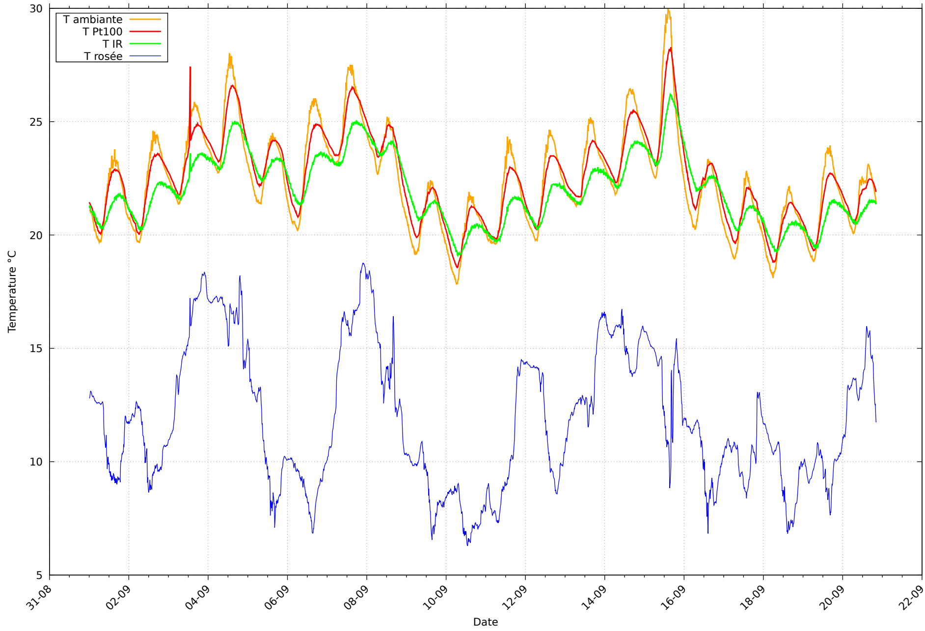
Température et rosée au 20/09/2026 pour RHT11
