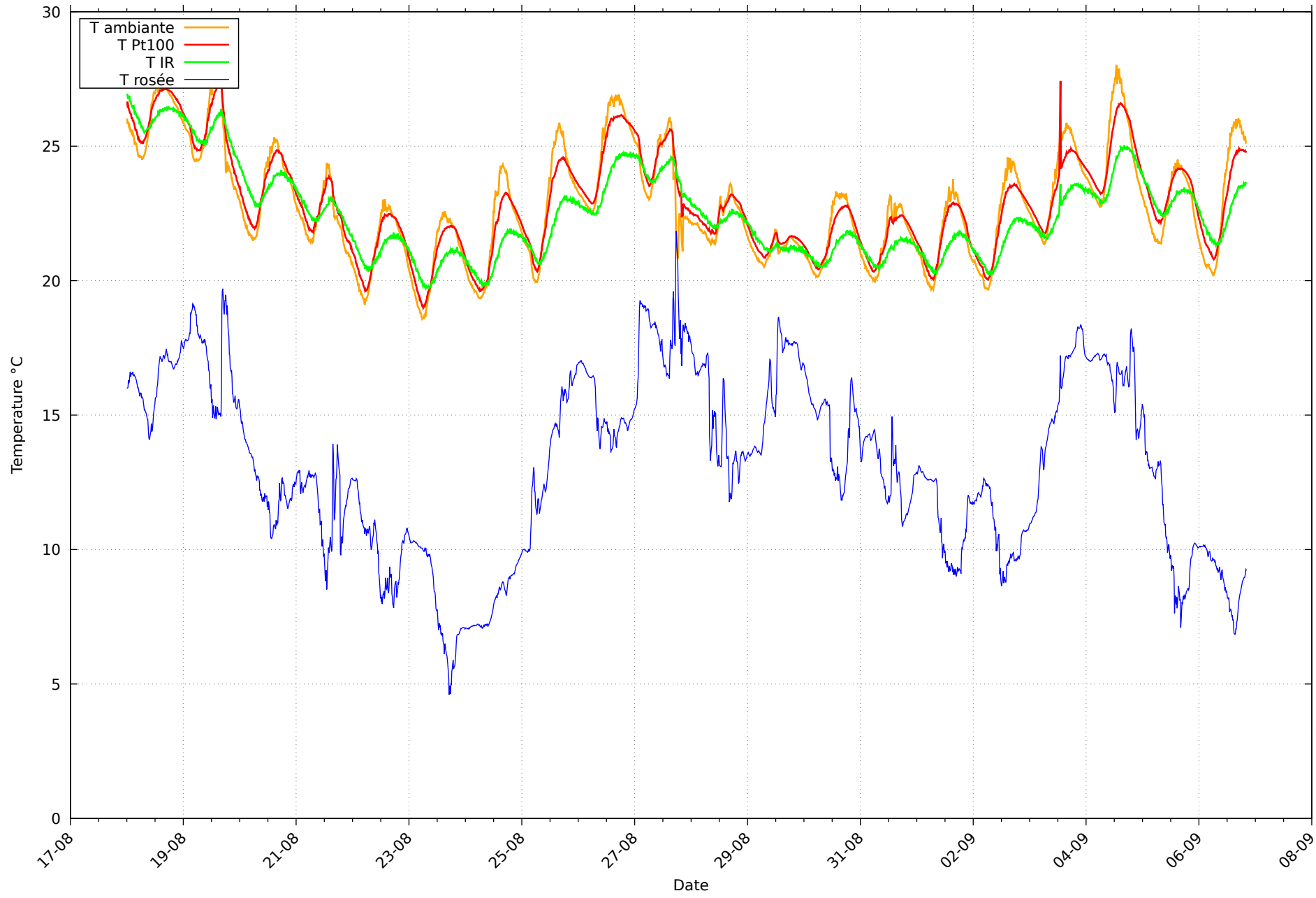
Température et rosée au 06/09/2026 pour RHT11
