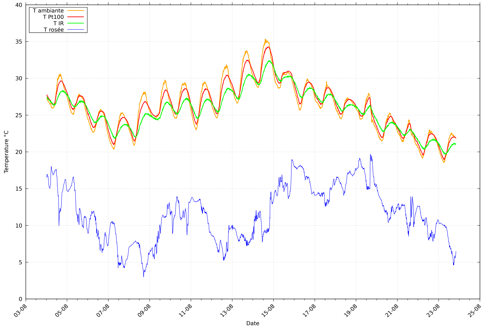
Température et rosée au 23/08/2026 pour RHT11
