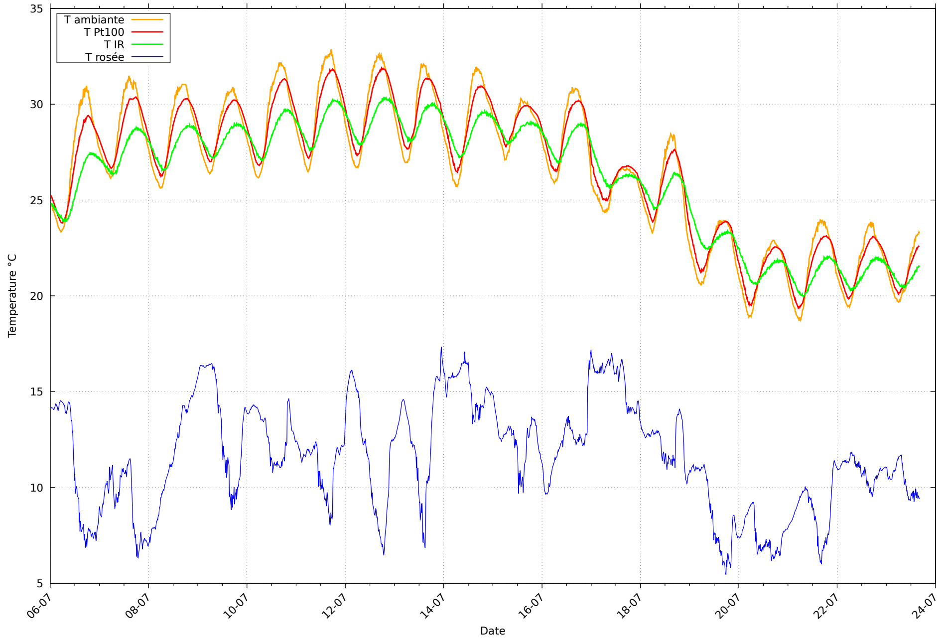
Température et rosée au 26/07/2026 pour RHT11
