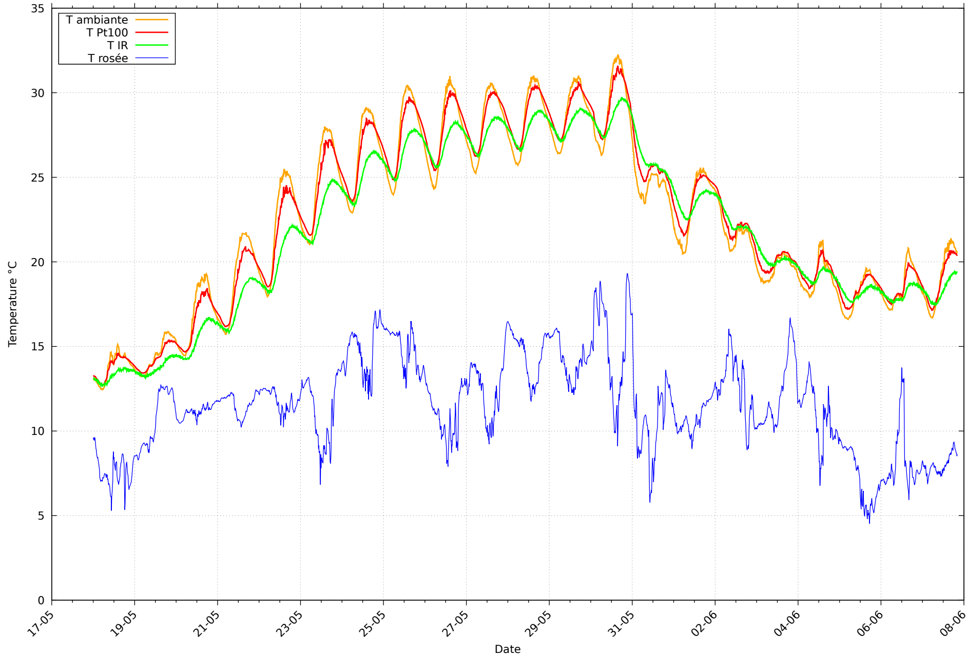
Température et rosée au 07/06/2026 pour RHT11
