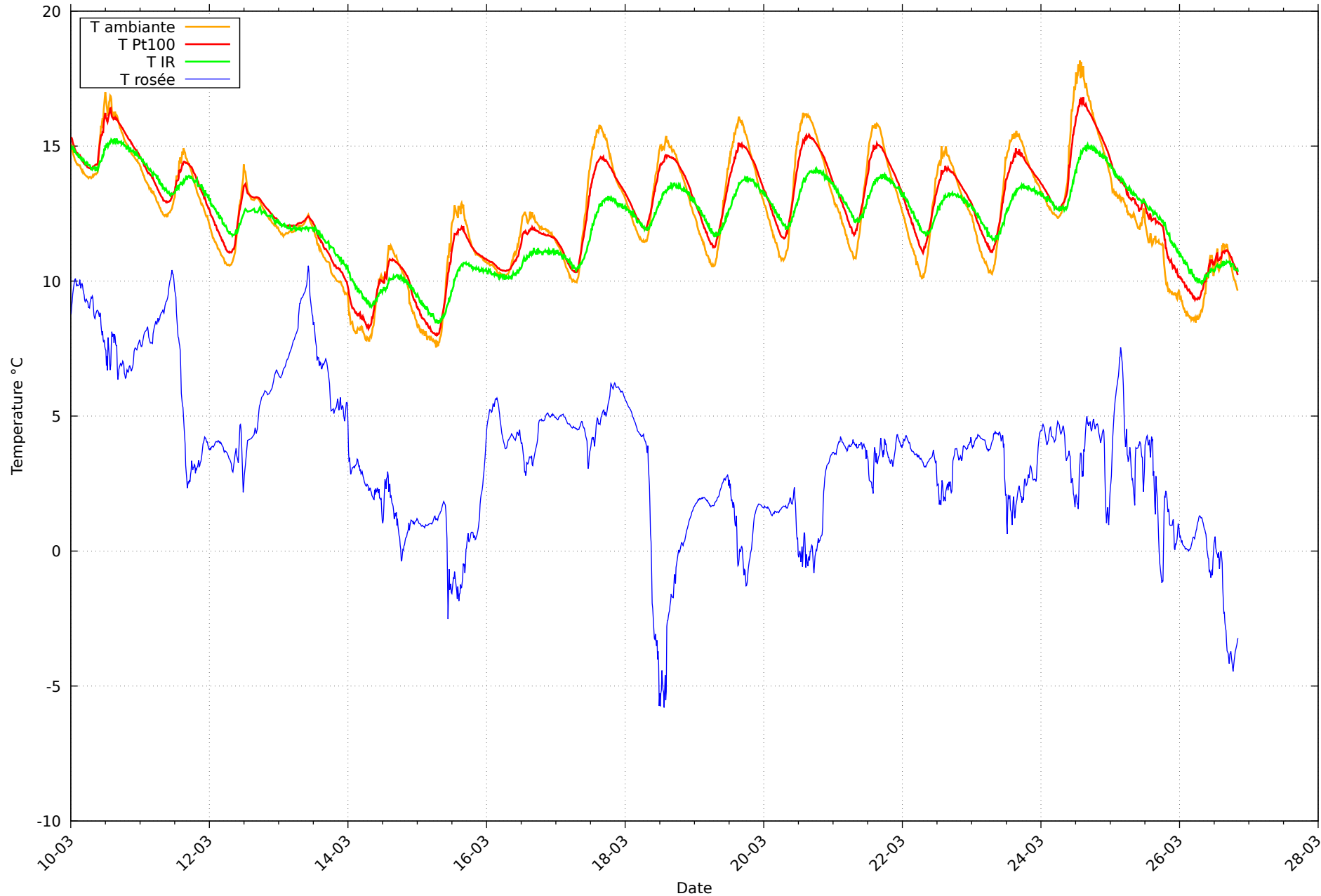
Température et rosée au 29/03/2026 pour RHT11
