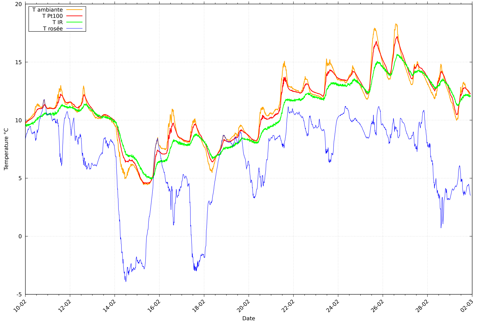
Température et rosée au 01/03/2026 pour RHT11
