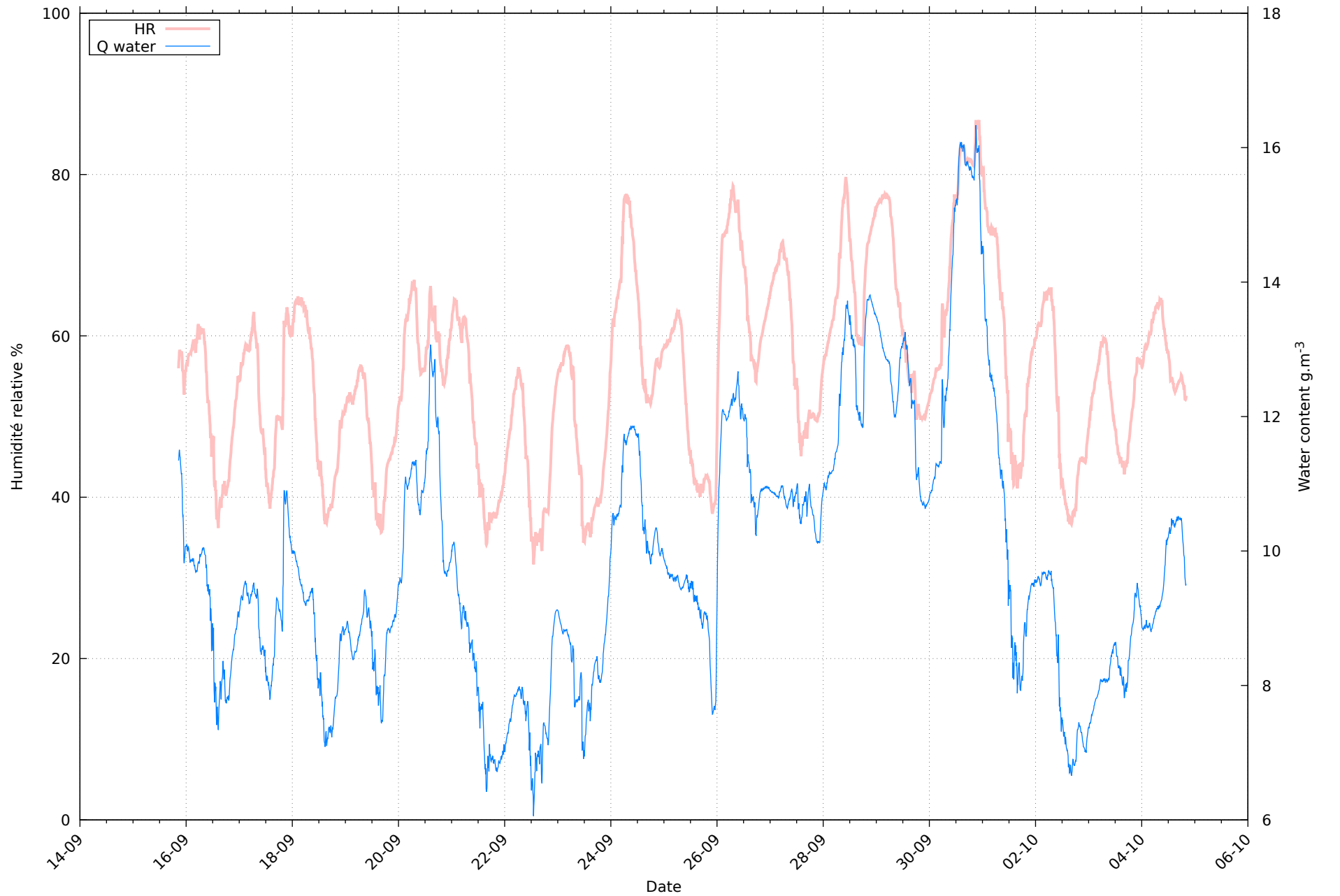
Humidité au 04/10/2026 pour RHT10
