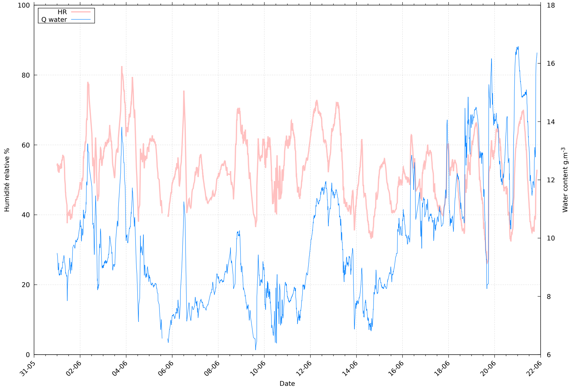
Humidité au 21/06/2026 pour RHT10
