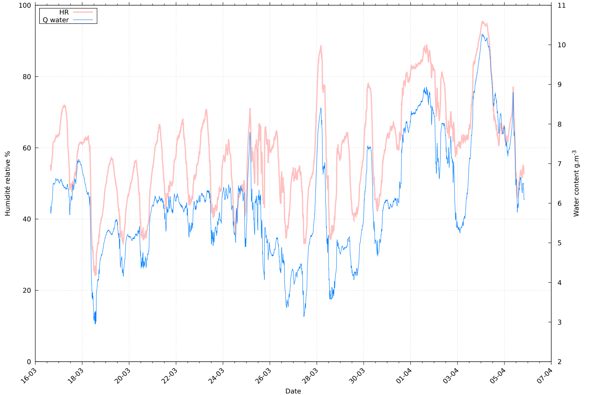
Humidité au 05/04/2026 pour RHT10
