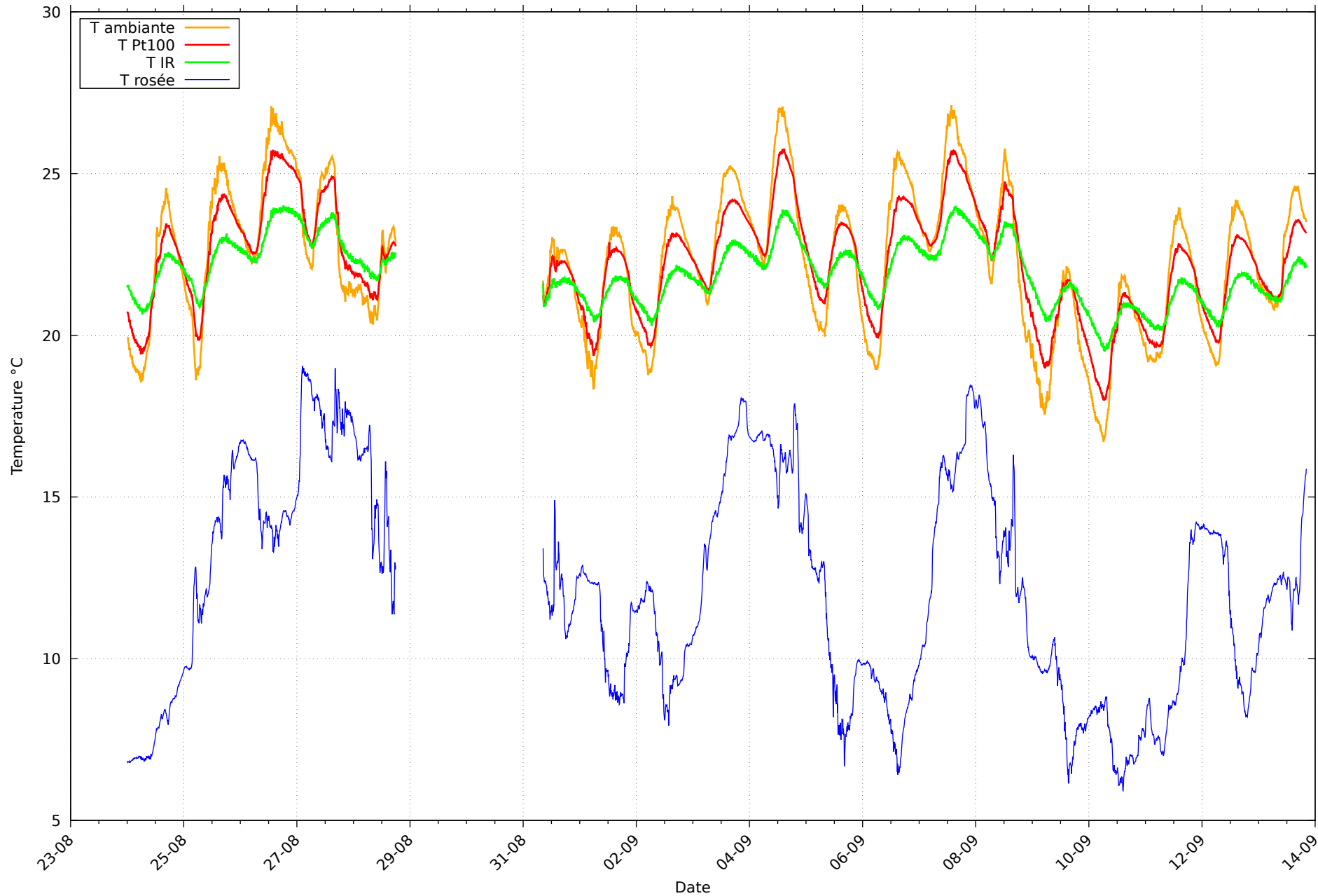
Température et rosée au 13/09/2026 pour RHT10
