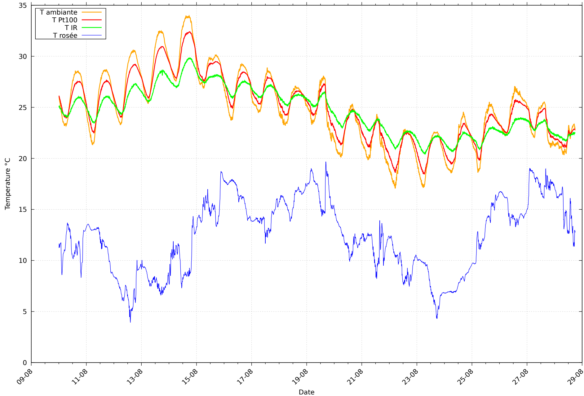
Température et rosée au 30/08/2026 pour RHT10
