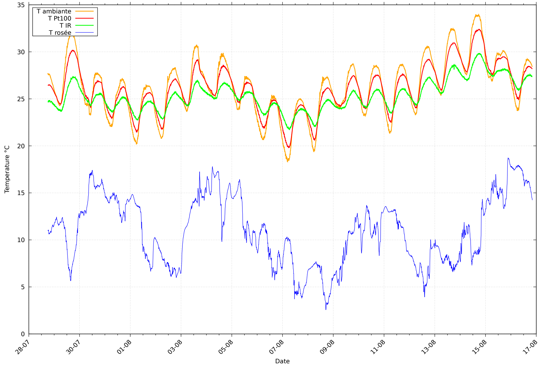
Température et rosée au 16/08/2026 pour RHT10
