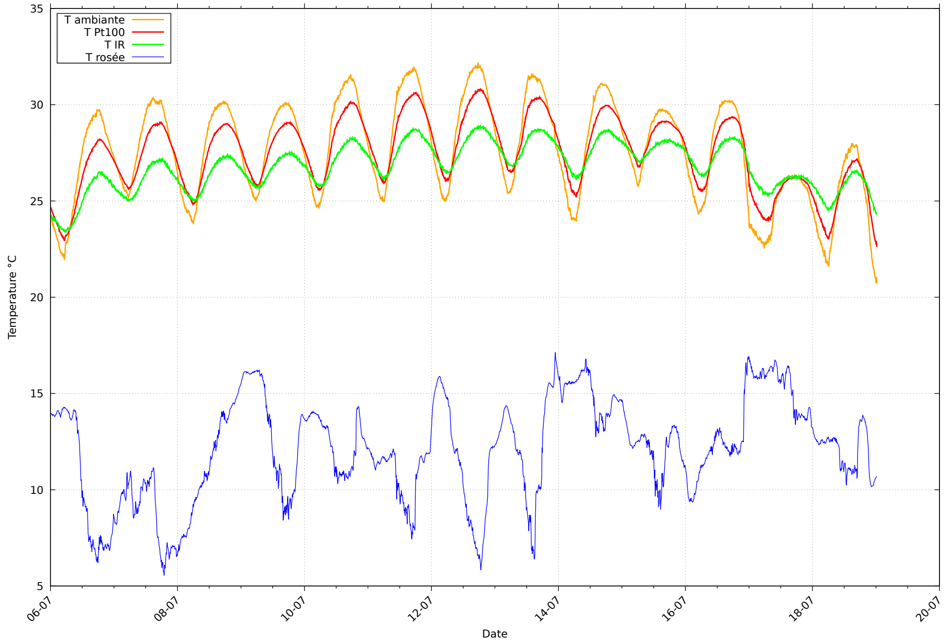
Température et rosée au 26/07/2026 pour RHT10
