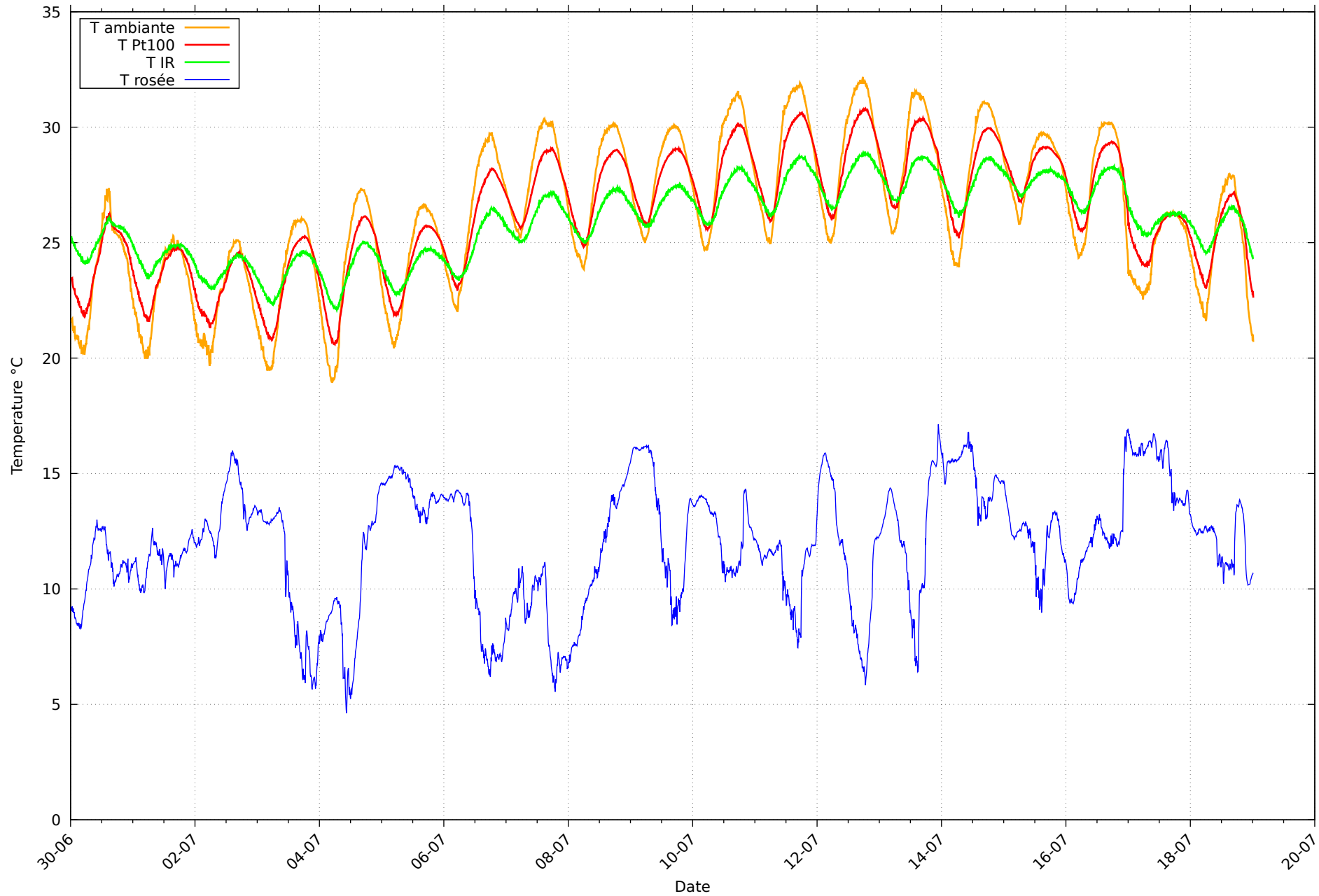
Température et rosée au 19/07/2026 pour RHT10
