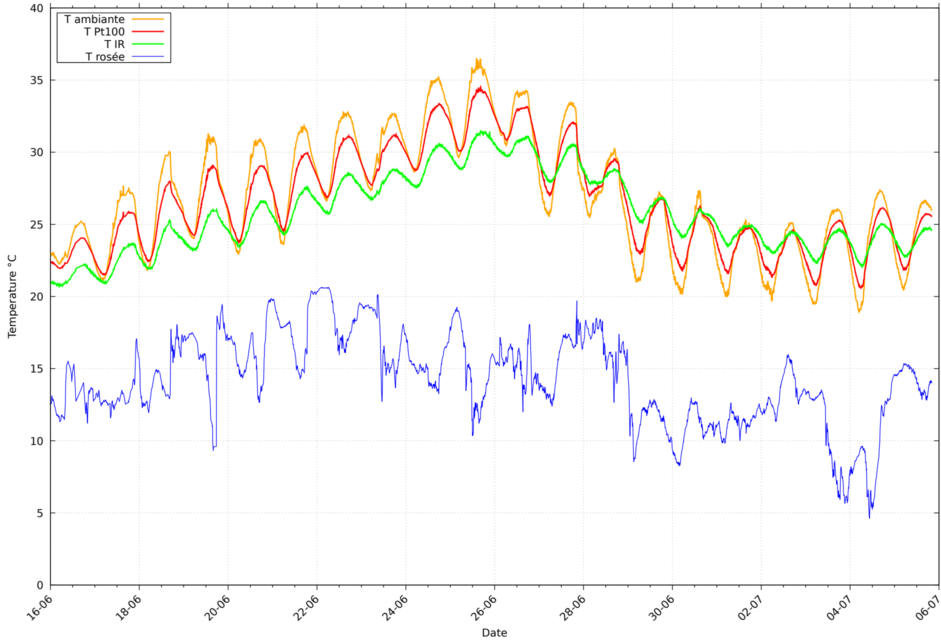
Température et rosée au 05/07/2026 pour RHT10
